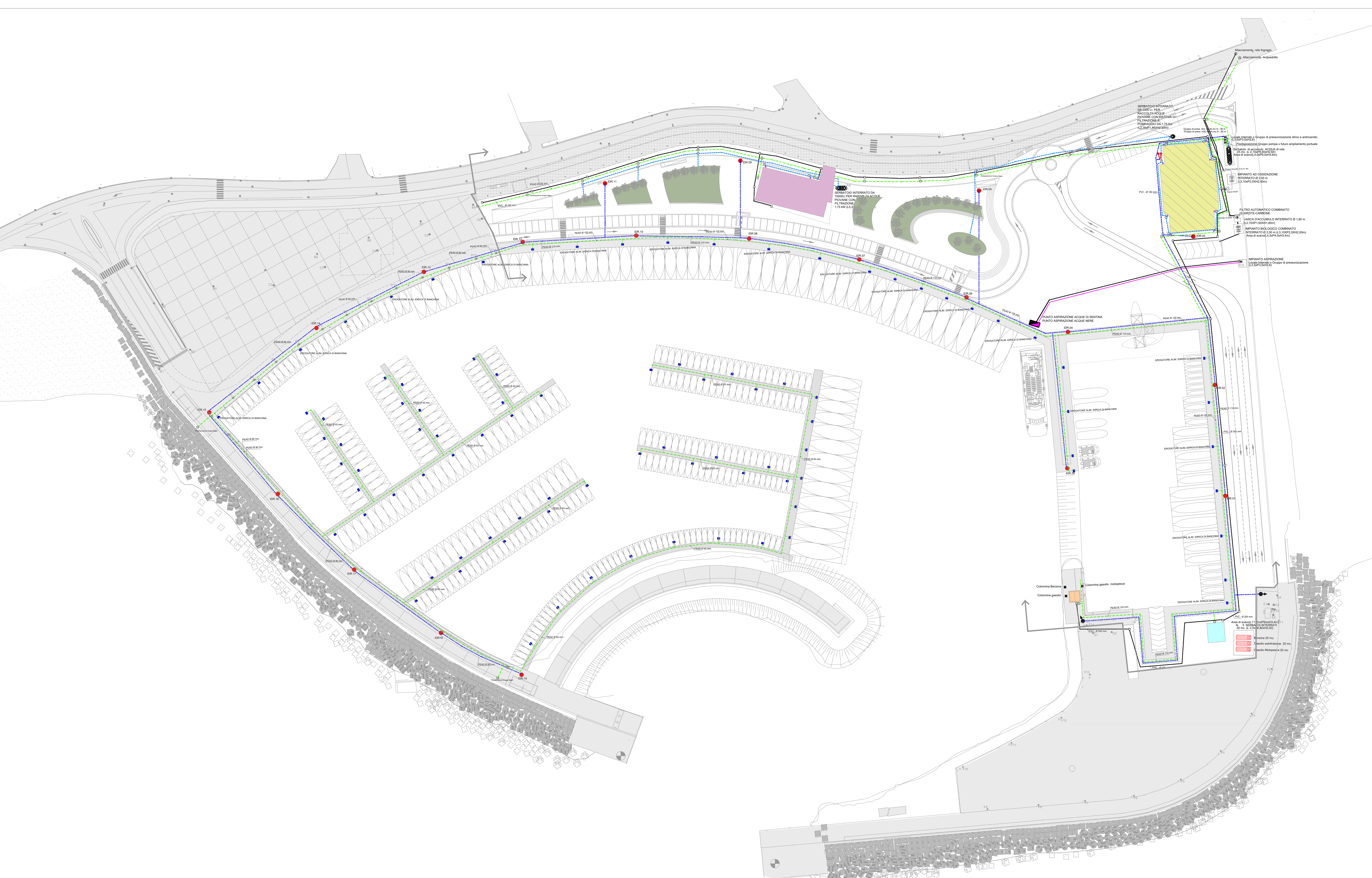
1 Planimetria generale - Distribuzione Generale 1:500
