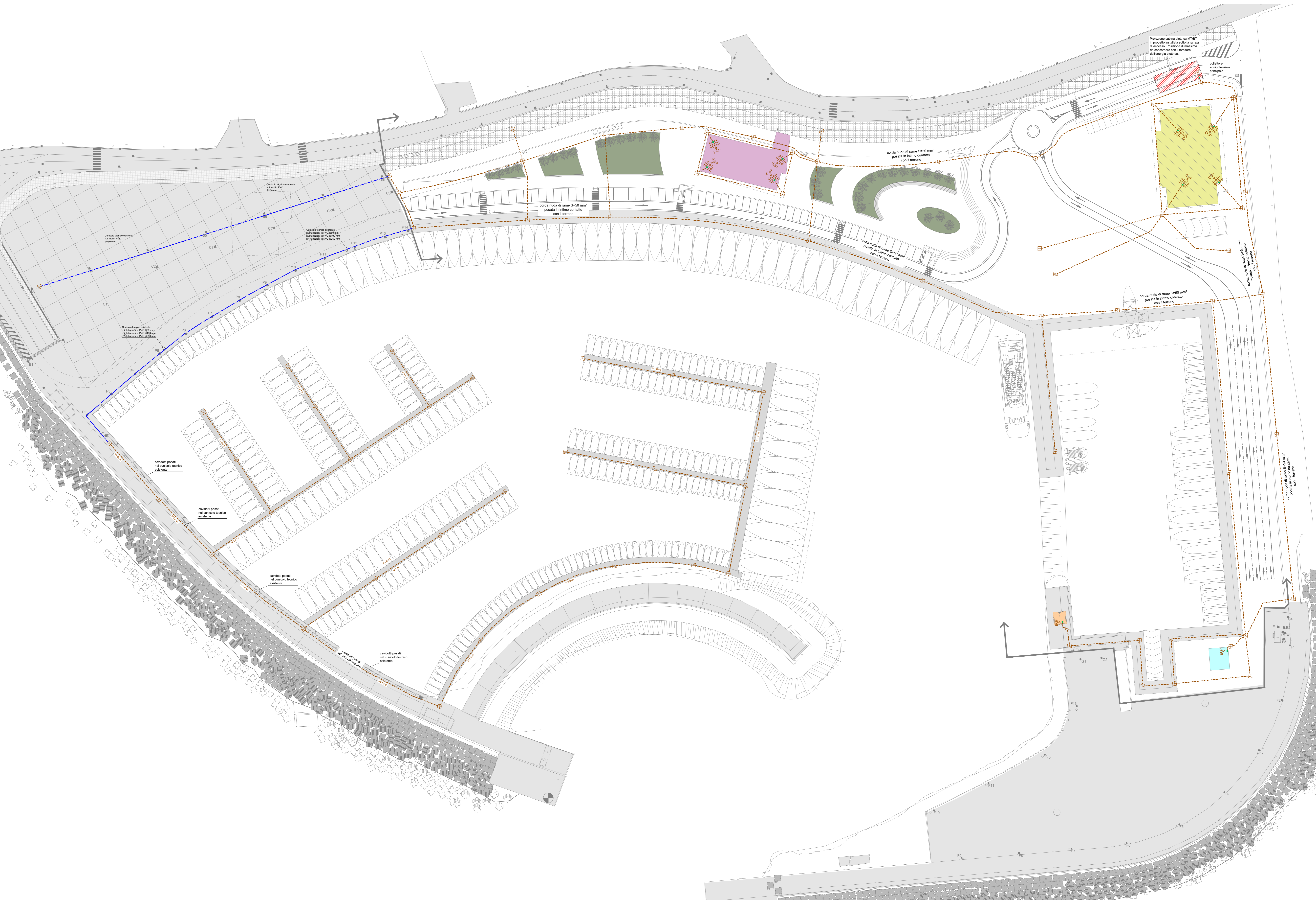
1 Planimetria generale 1:500
