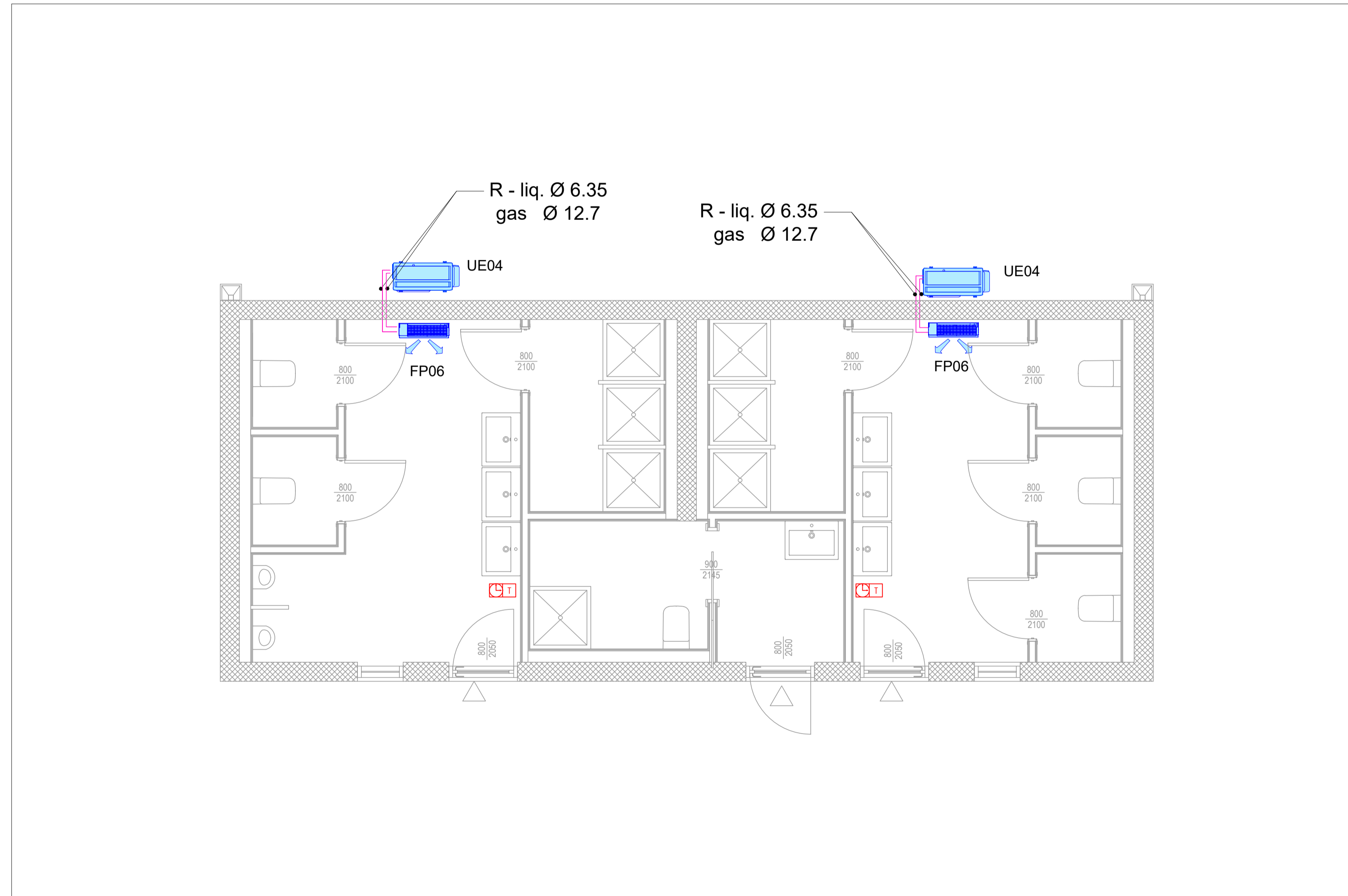
1 Blocco bagno tipo- impianto di condizionamento 1:40
