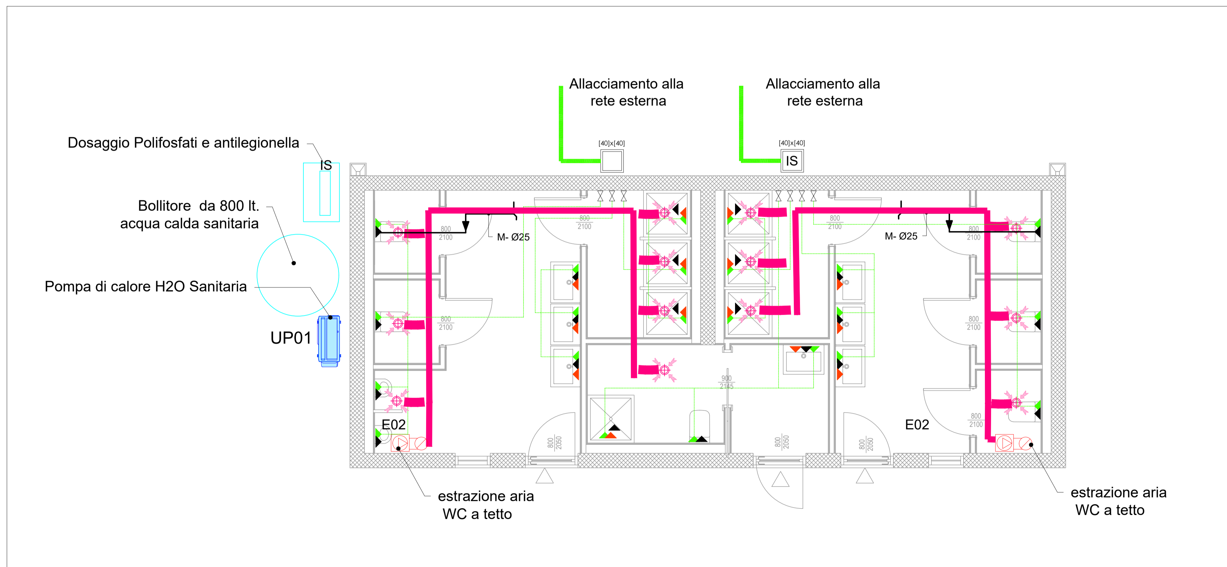
1 Blocco bagno tipo- impianto idrico e scarico 1:40
