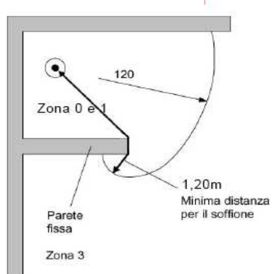
f) Doccia senza piatto con parete fissa
