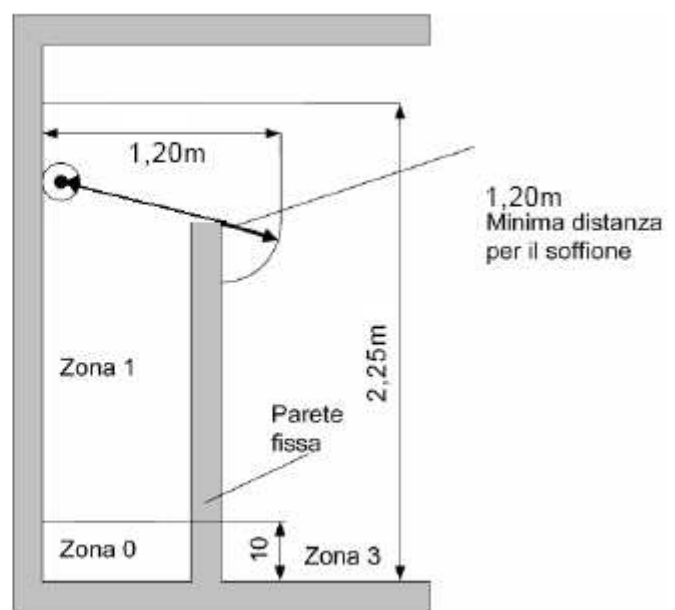
d) 2) Alzata (con parete fissa)
