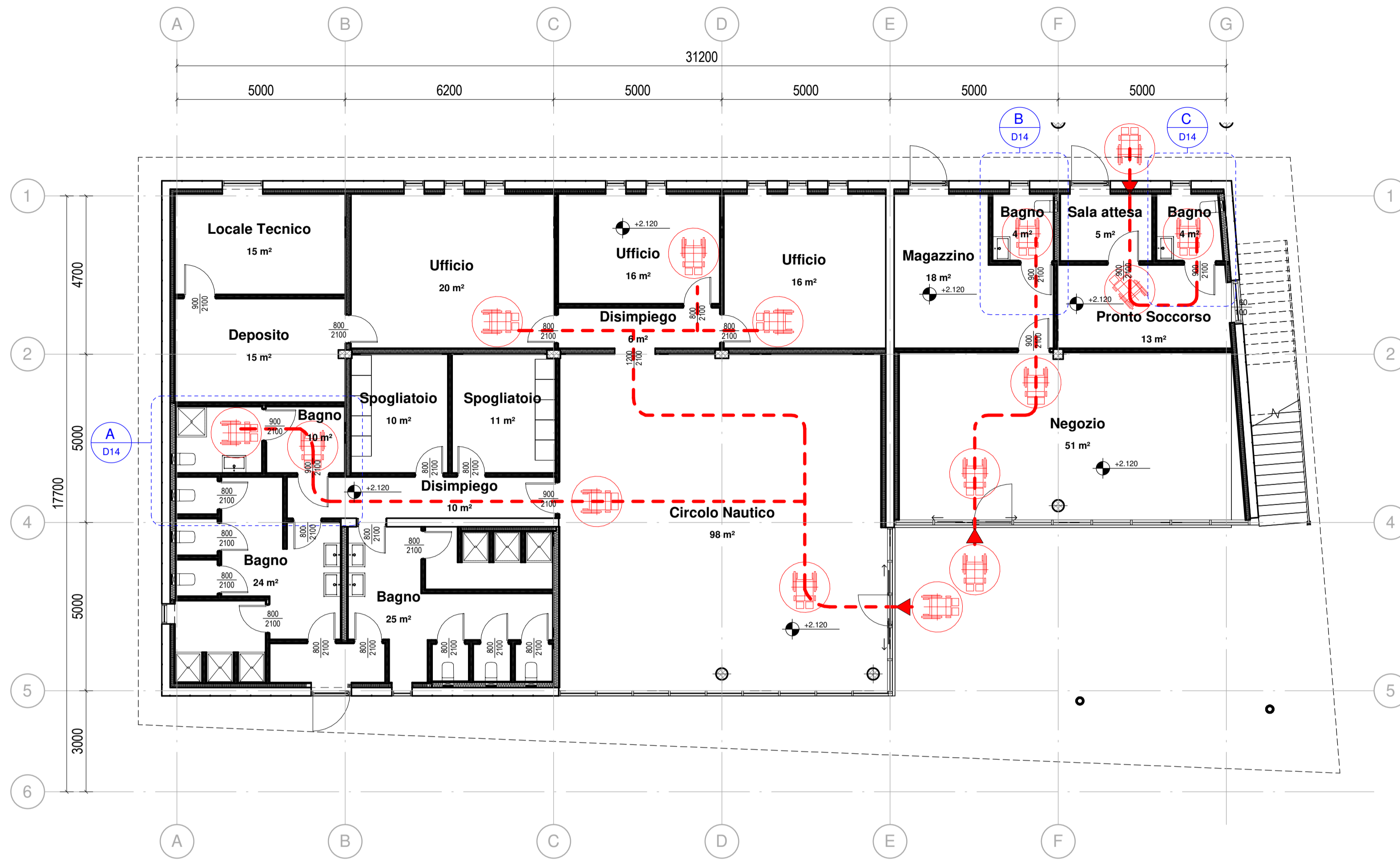
Pianta Scale 1 : 100
