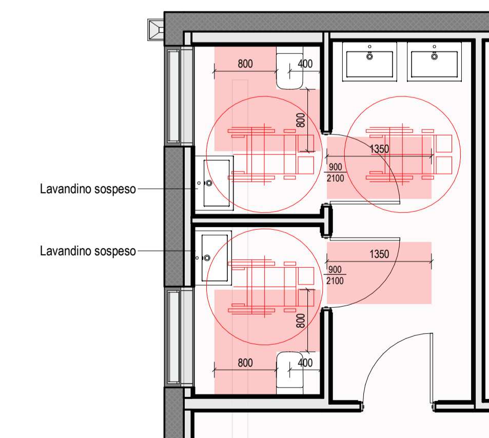
Servizi Igienici A Scale 1 : 50
