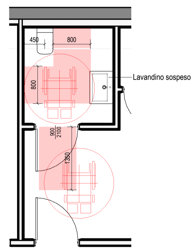
Servizi Igienici B Scale 1 : 50
