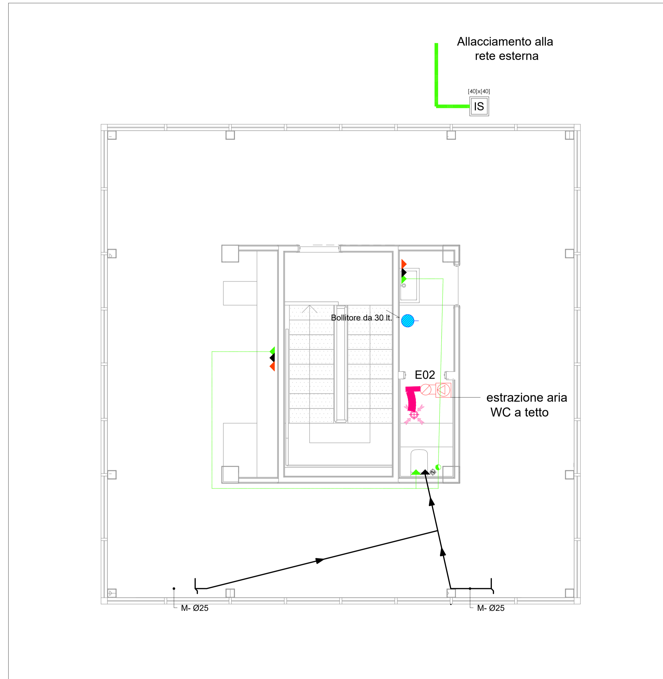
1 F - Planimetria Torre di controllo - impianto idrico e scarico 1:40
