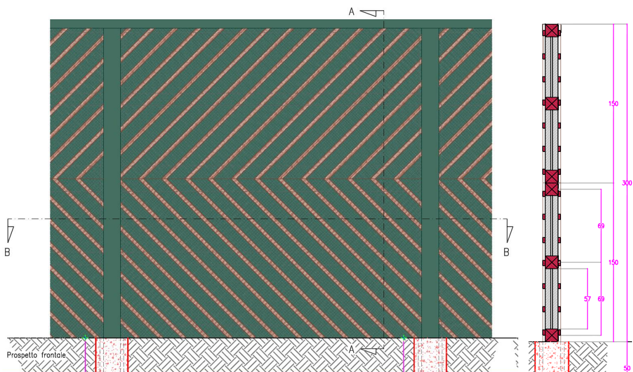
FIGURA 2-9 –BARRIERA ACUSTICA IN LEGNO: VISTA PROSPETTICA E SEZIONE VERTICALE
