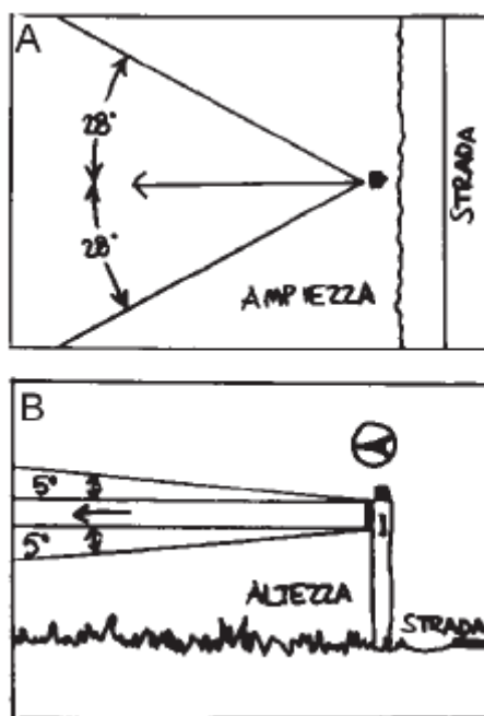
FIGURA 2-7- AMPIEZZA (A) ED ALTEZZA (B) DEL FASCIO DI LUCE RIFLESSA
