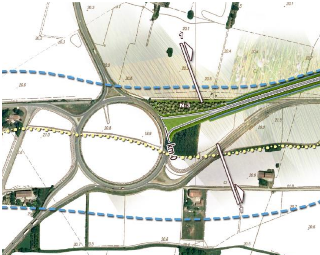
FIGURA 2-2 - TIPOLOGIA N3 IN PROSSIMITA' DELLA ROTATORIA A NORD DEL CAVO TAGLIATA
