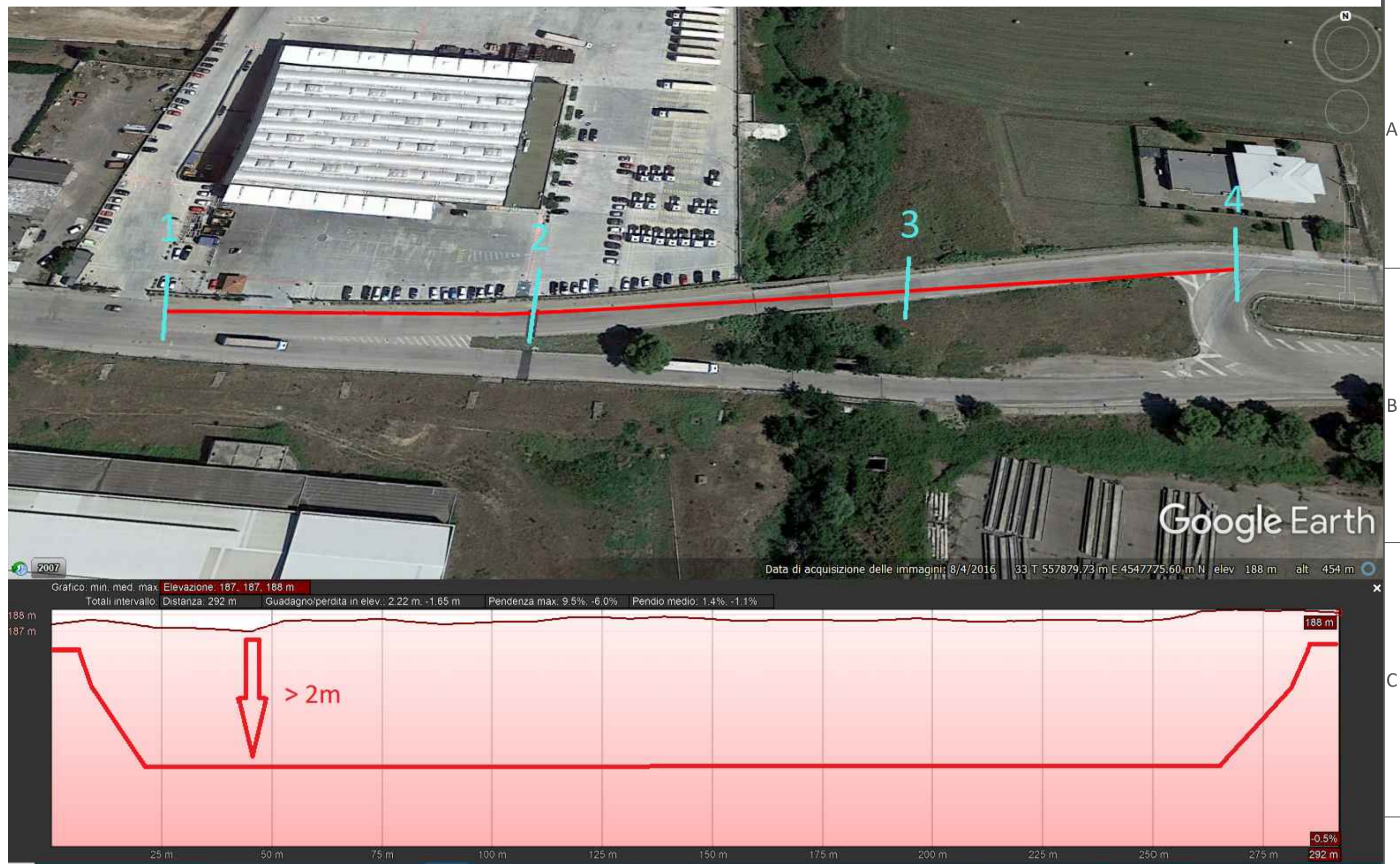
STRALCIO DEL PROFILO LONGITUDINALE DELLA T.O.C. VALLONE CASELLA
