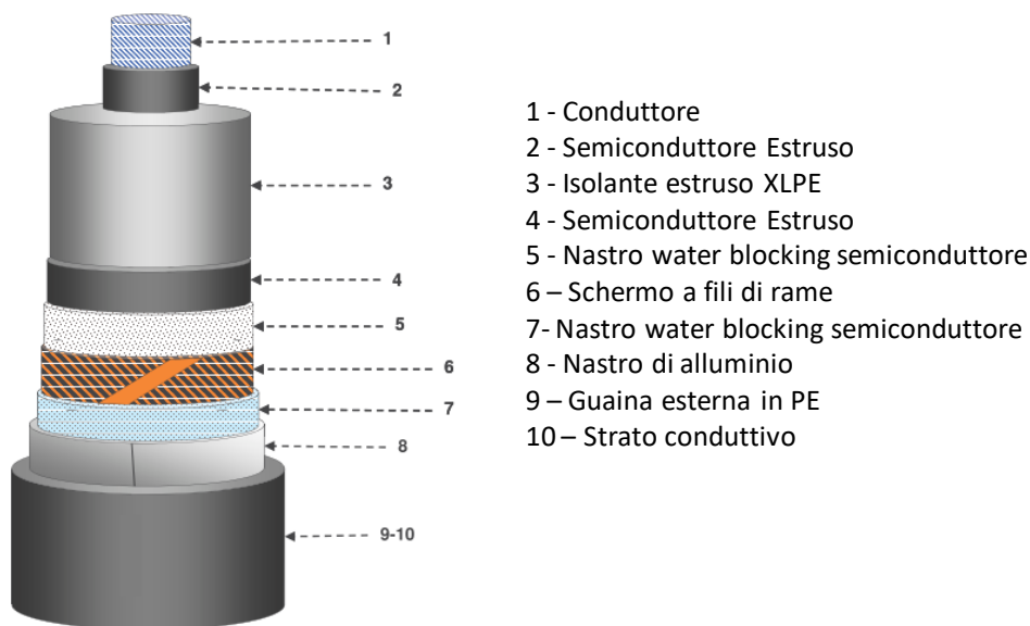
Figura 5.1 - Cavo AT 150 kV tipo ARE4H1H5E 87/150kV
