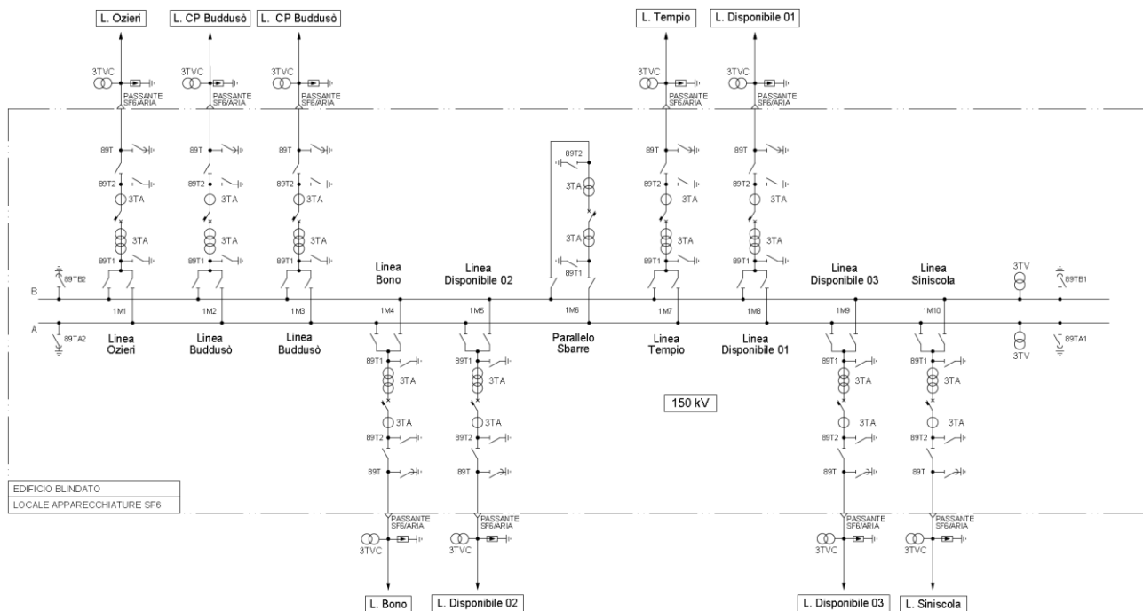
Figura 3.1 – Schema unifilare nuova SE Terna “Buddusò”
