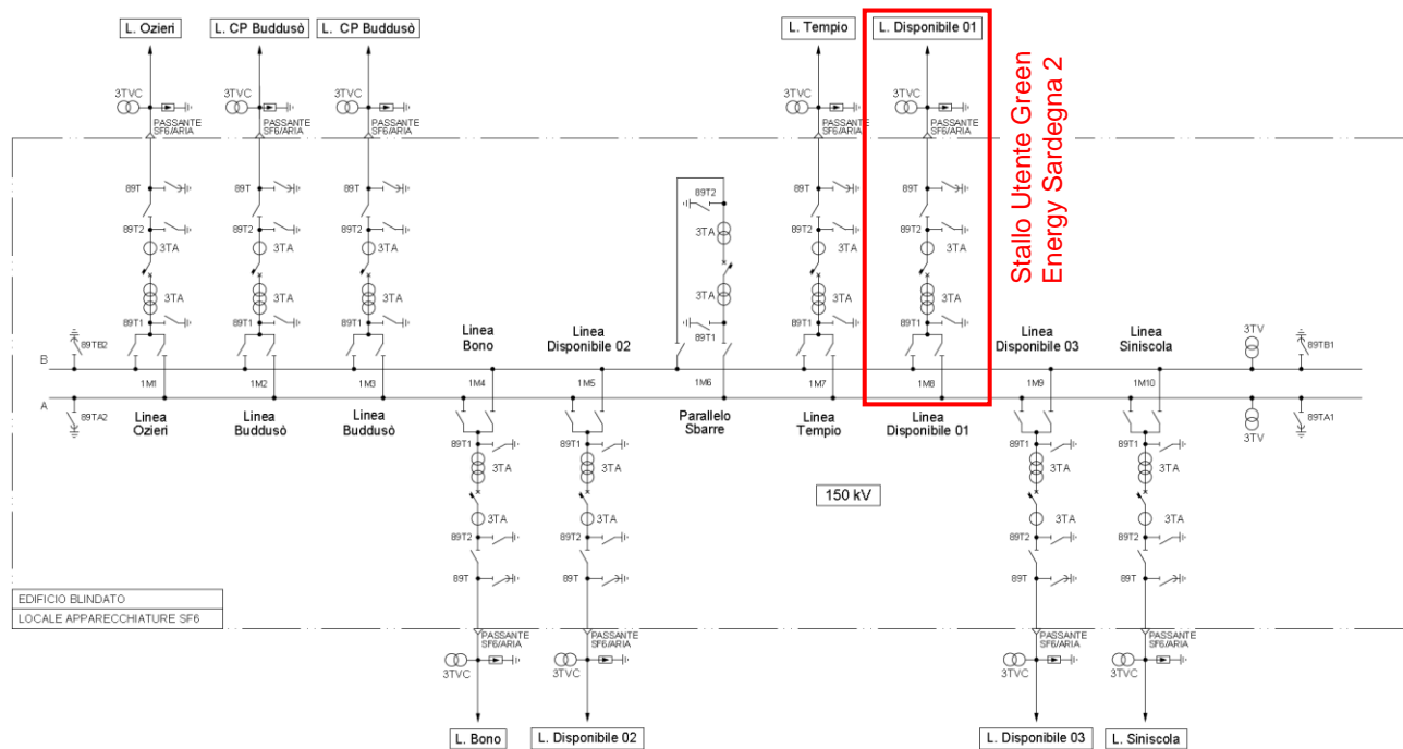
Figura 4.1 – Schema unifilare nuova SE Terna “Buddusò” – Ipotesi Stallo Utente Green Energy Sardegna 2
