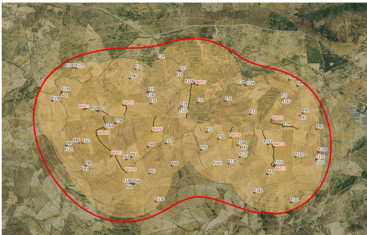
Figura 2.5 – Campo sonoro generato dall’impianto. In rosso l’isofonica dei 33 dBA, attestata ad una distanza indicativa di 1.000 m dalle postazioni eoliche in progetto
