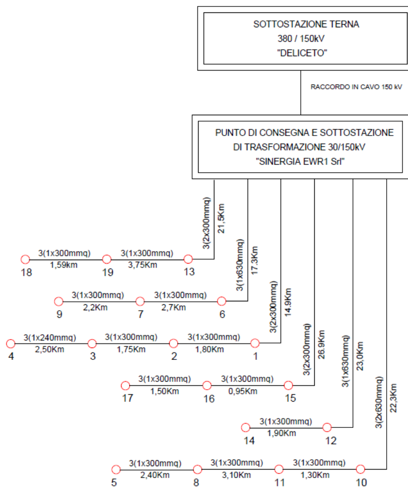
Schema elettrico unifilare WTG
