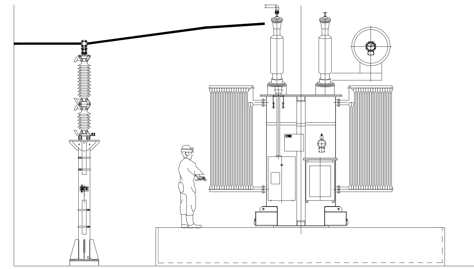
PARTICOLARE TRAFÒ Ingrandimento vista
