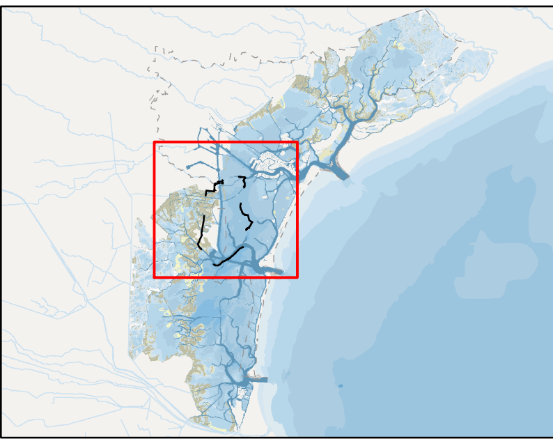
Cartografia progetto definitivo interventi per la protezione e la conservazione dei fondali del canale Malamocco - Marghera da realizzarsi nelle relative aree di bordo - primo stralcio e Buffer di interferenza (fase di cantiere)
