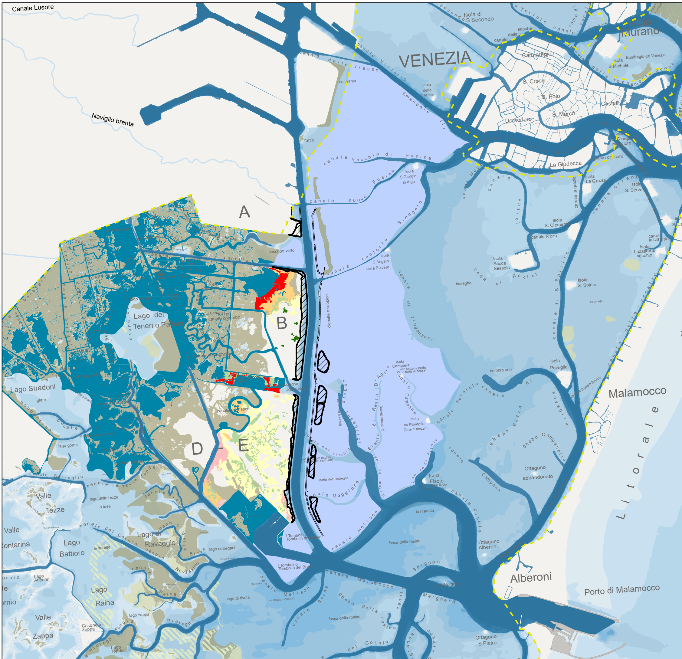
Cartografia progetto definitivo interventi per la protezione e la conservazione dei fondali del canale Malamocco - Marghera da realizzarsi nelle relative aree di bordo - primo stralcio e Buffer di interferenza (fase di cantiere)
