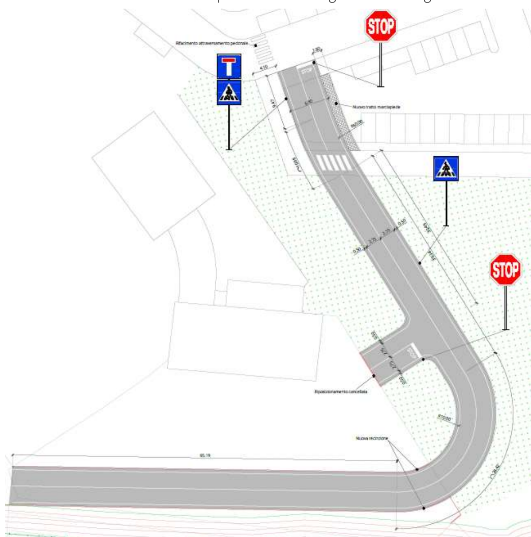
Figura 8: stato di progetto accesso km 150+900
