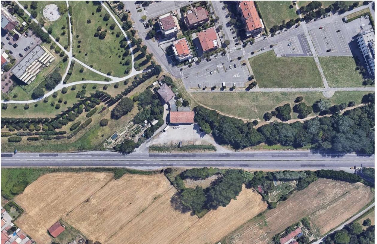
Figura 6: accessi km 150+860 e km 150+940 dir. Nord
