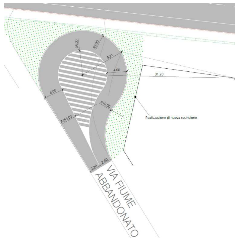
Figura 27: Stato di progetto viabilità secondaria km 150+650
