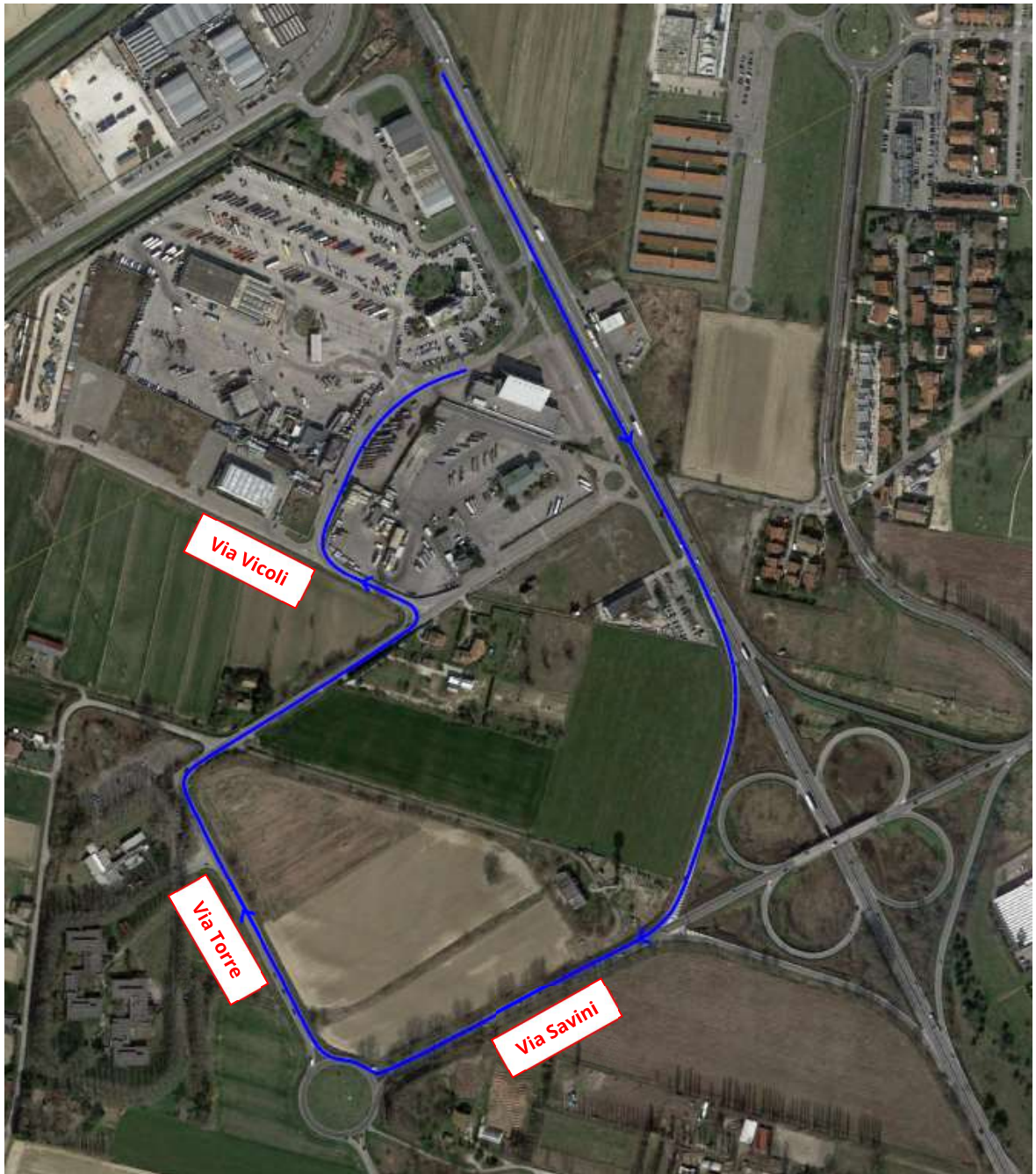
Figura 4: percorso alternativo accesso km 149+026 dir. Sud
