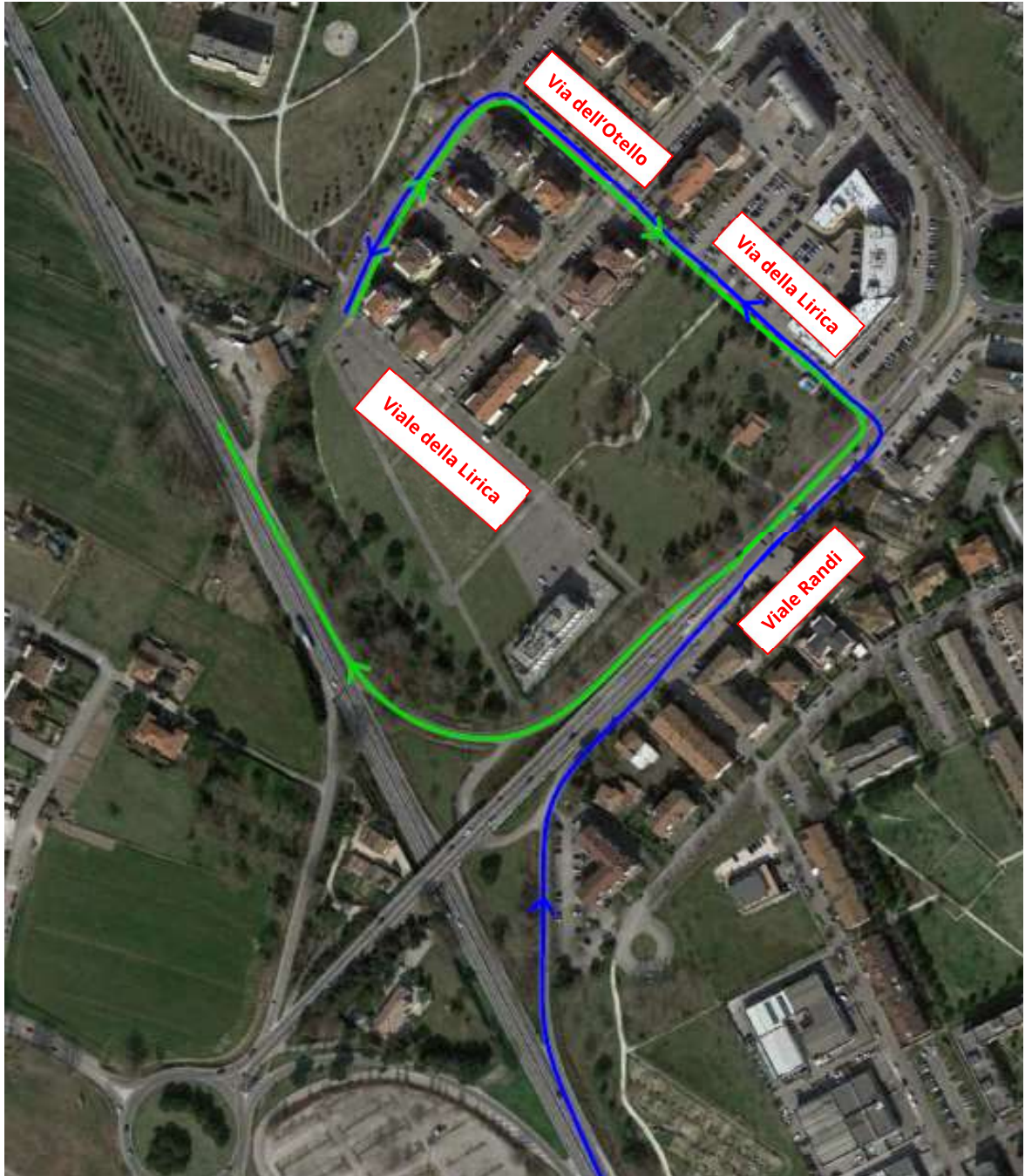
Figura 7: percorso alternativo accessi km 150+860 e km 150+940 dir. Nord
