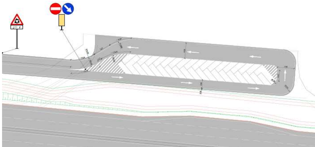
Figura 21: Stato di progetto accesso da km 153+650 a km 154+000
