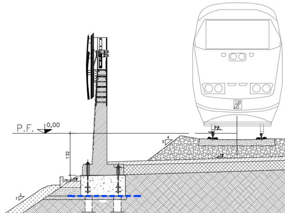
Figura 9 - Sezione considerata per le verifiche
