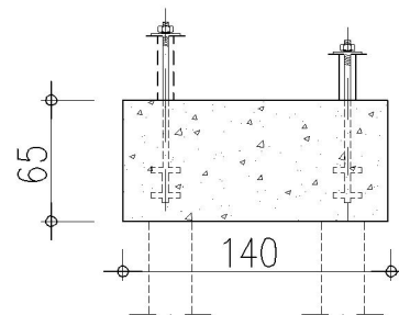
Figura 3 – Tipologico cordolo di fondazione
