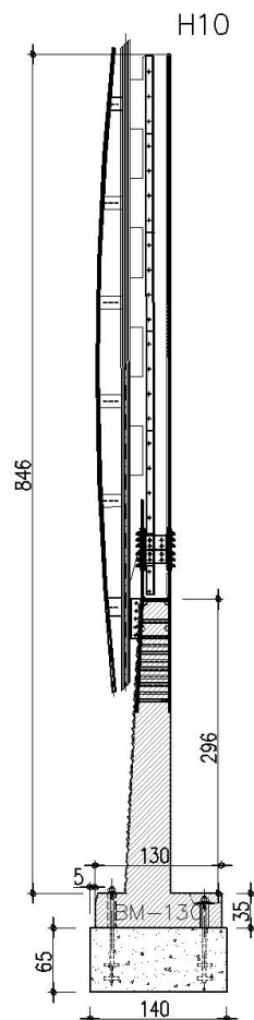
Figura 2 – Tipologico BA H10
