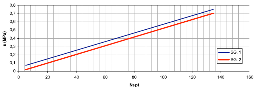
Figura 10 - Abaco per la determinazione di s per sabbie e ghiaie
