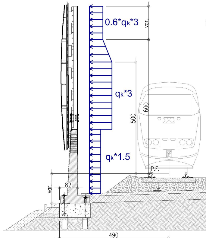
Figura 8 - Distribuzione delle pressioni sull'altezza della barriera
