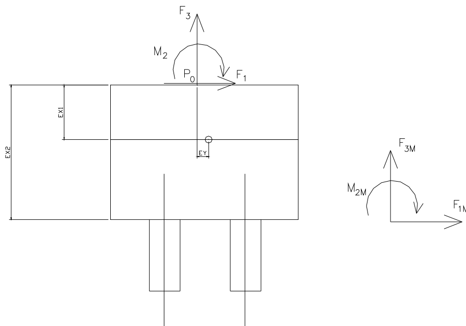
Figura 4 - Sistemi di riferimento e punti di verifica
