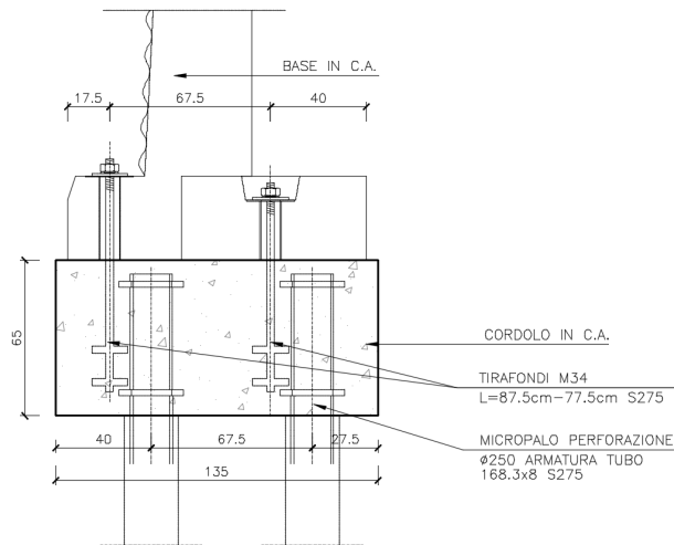
Figura 2 – Dettaglio fondazione modulo BS125-450
