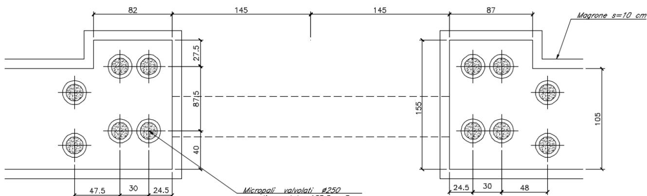
Figura 3 – Pianta fondazione modulo BS145-450
