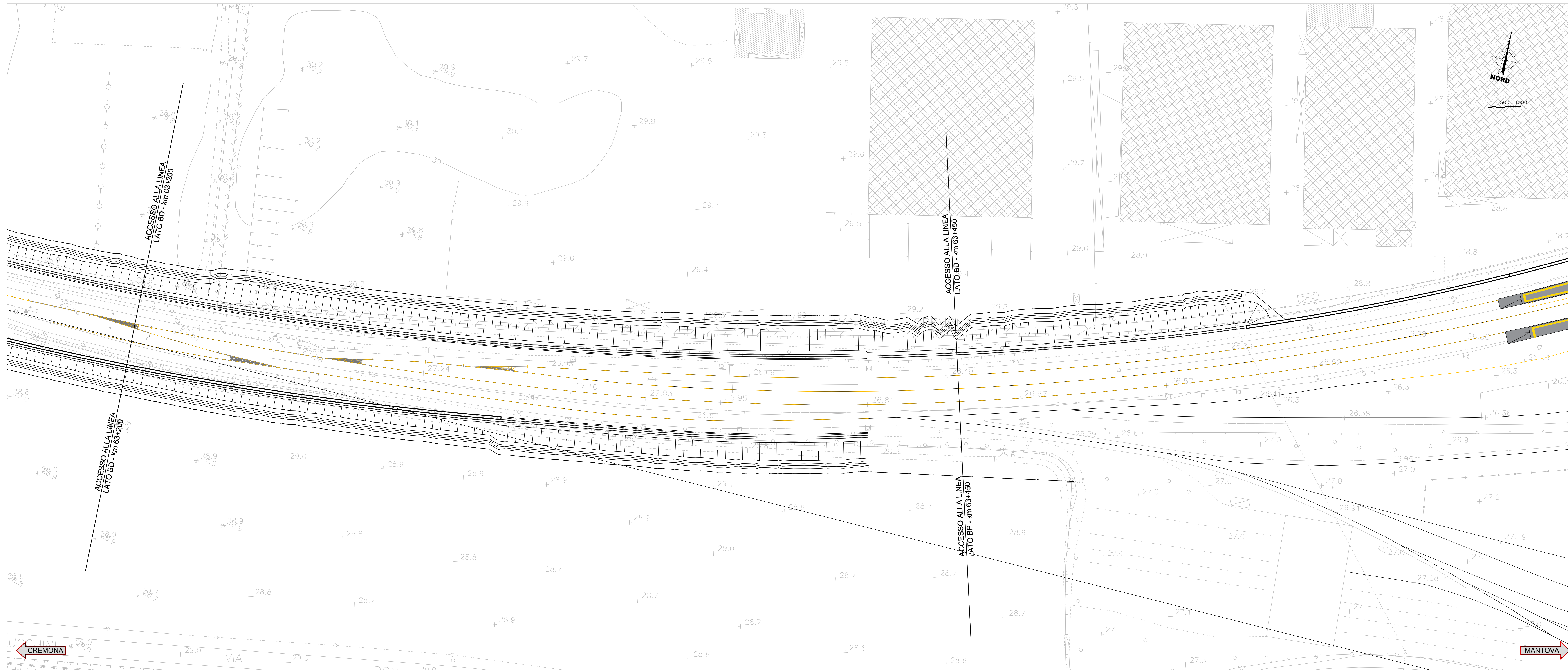
PIANTA - Scala 1:500
