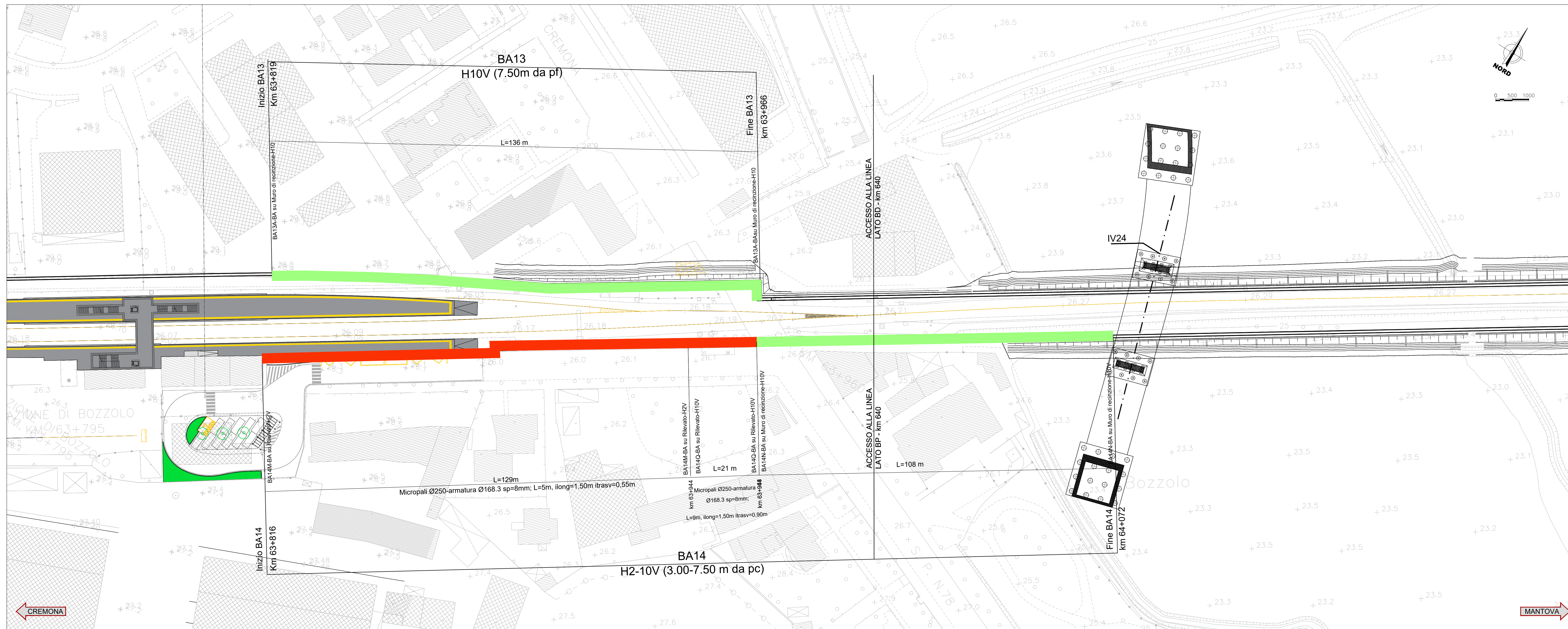
PIANTA - Scala 1:500
