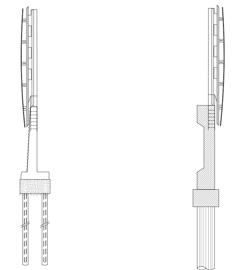
BARRIERA SU RILEVATO / BARRIERA SU OPERA DI RECINZIONE Scala 1:100
