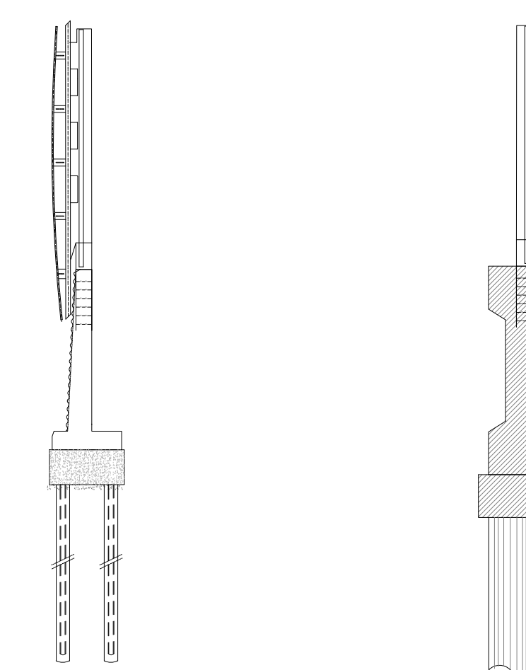
BARRIERA SU RILEVATO BARRIERA SU OPERA DI RECINZIONE Scala 1:100
