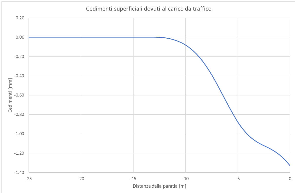
Figura 13 – Cedimenti indotti dal carico ferroviario
