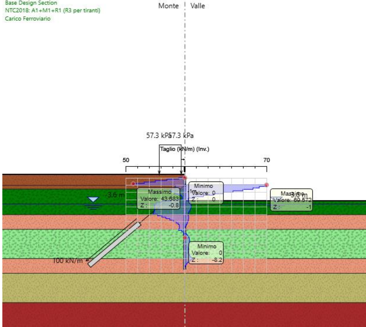
Figura 4 – Modello SLU: Involuppo Diagramma del Taglio
