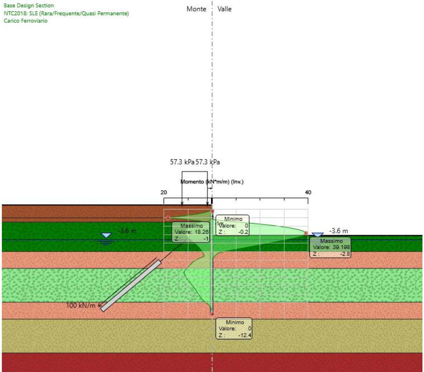
Figura 2 – Modello SLE: Involuppo Diagramma del Momento
