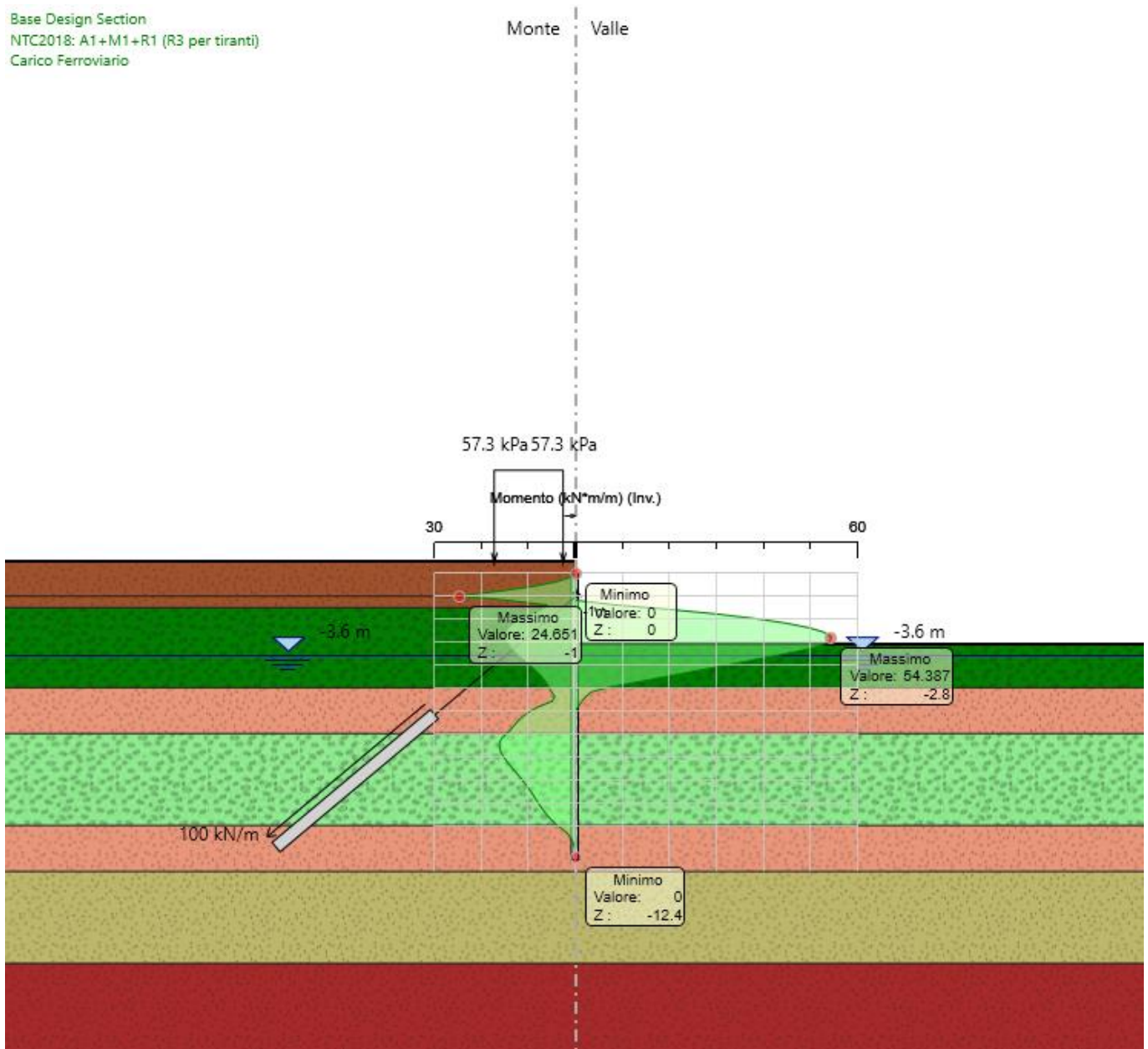
Figura 3 – Modello SLU: Involuppo Diagramma del Momento
