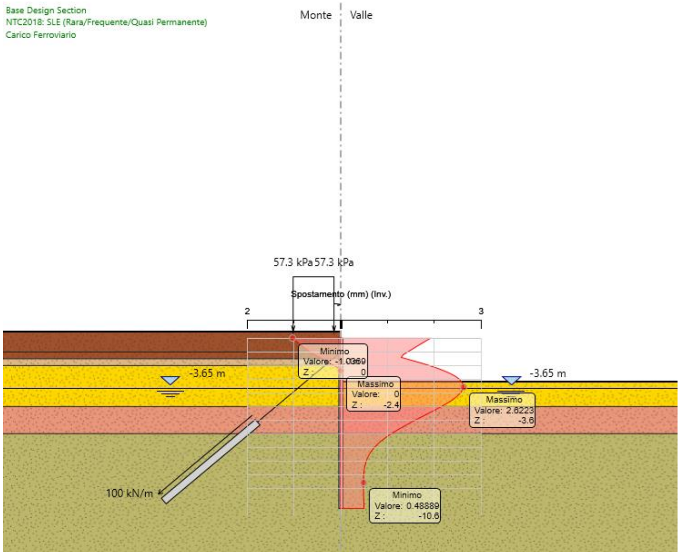
Figura 5 – Modello SLE: Inviluppo degli spostamenti
