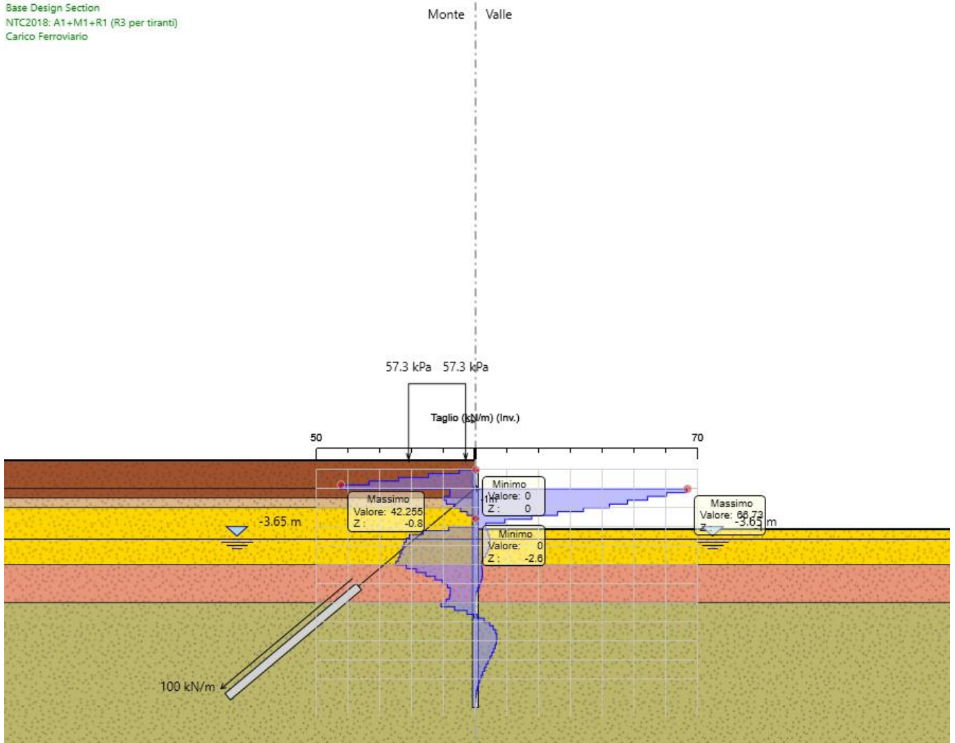
Figura 4 – Modello SLU: Involuppo Diagramma del Taglio
