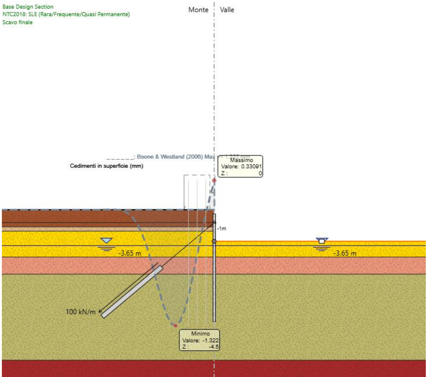
Figura 12 – Cedimenti superficiali – Fase: raggiungimento fondo scavo
