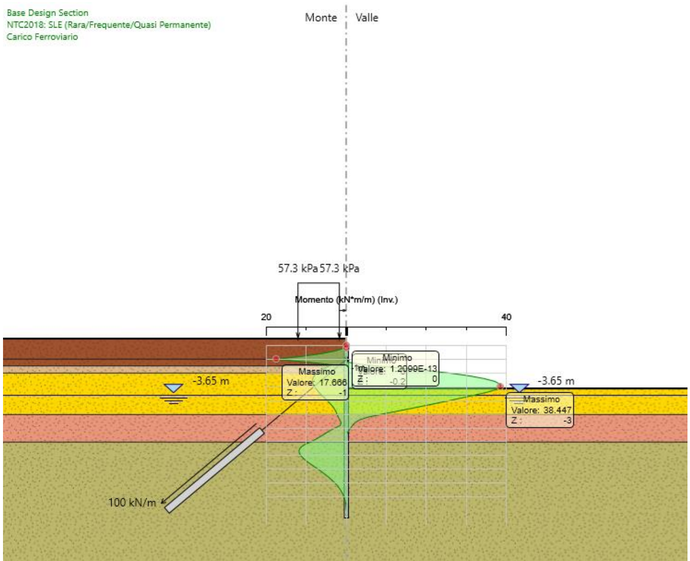
Figura 2 – Modello SLE: Involuppo Diagramma del Momento
