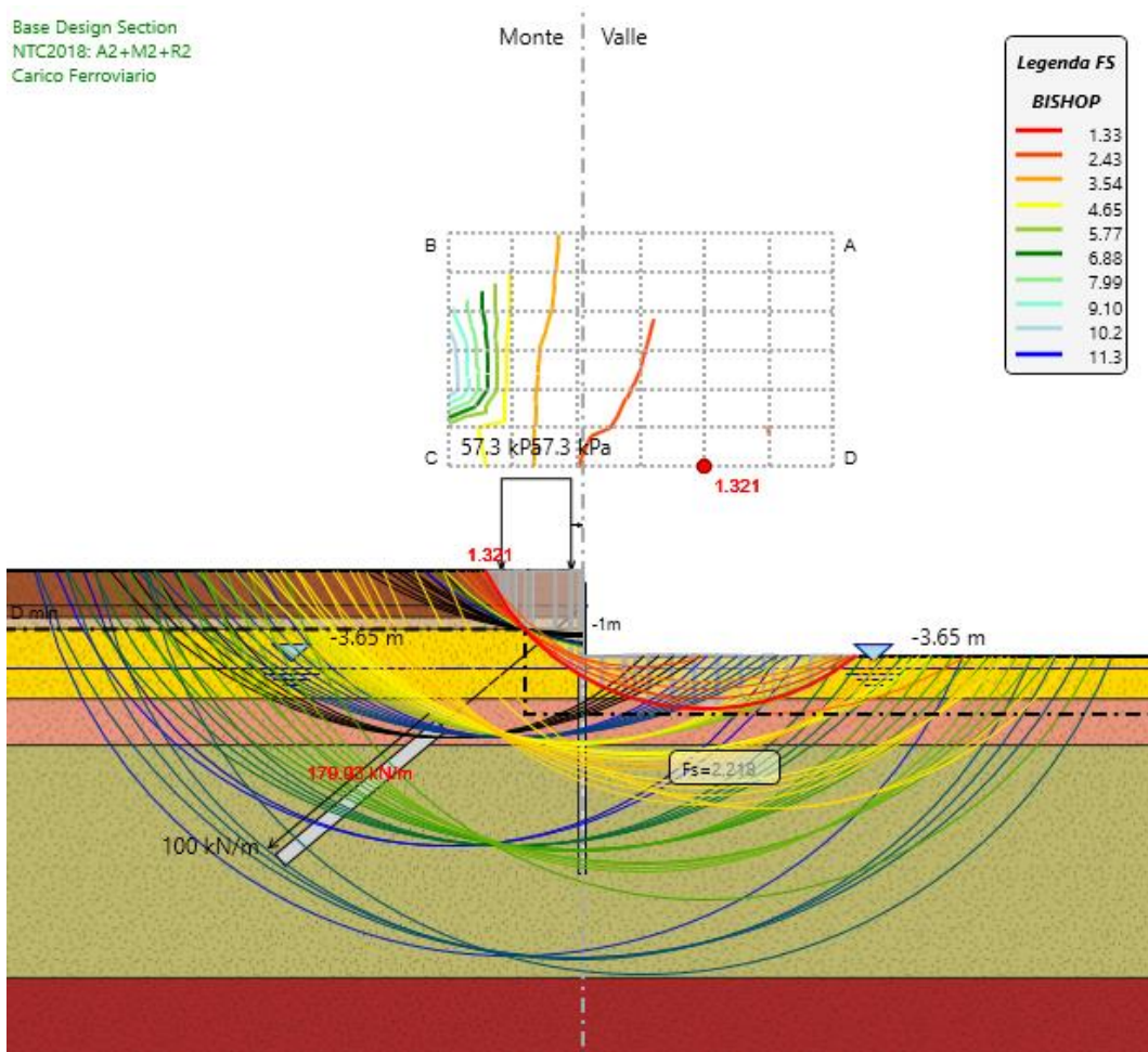
Figura 7 – Risultati dell'analisi di stabilità globale
