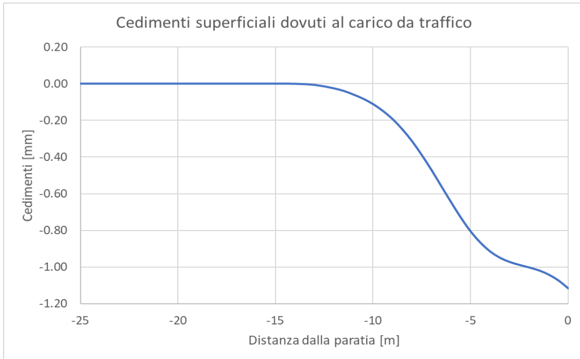
Figura 13 – Cedimenti indotti dal carico ferroviario
