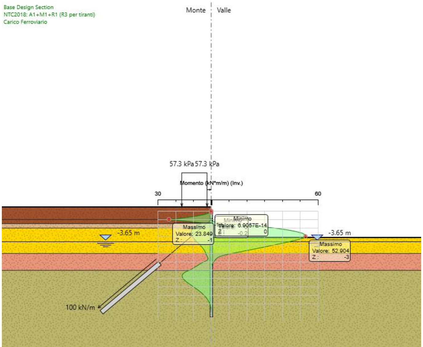
Figura 3 – Modello SLU: Involuppo Diagramma del Momento
