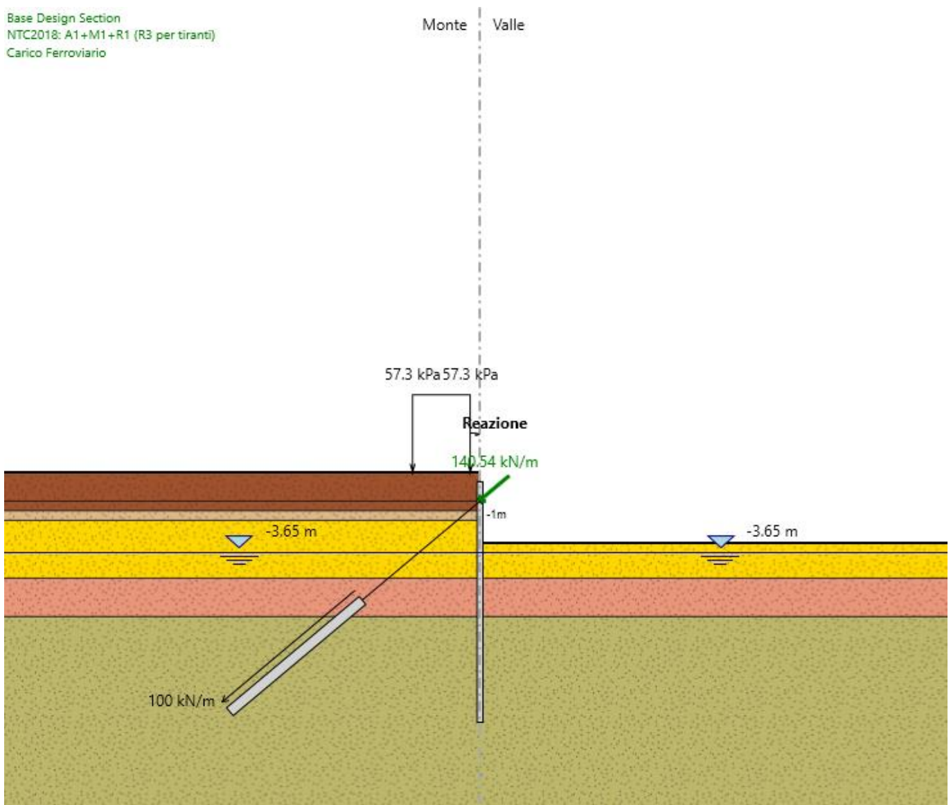
Figura 6 – Modello SLU: Involuppo Sollecitazioni nei Tiranti
