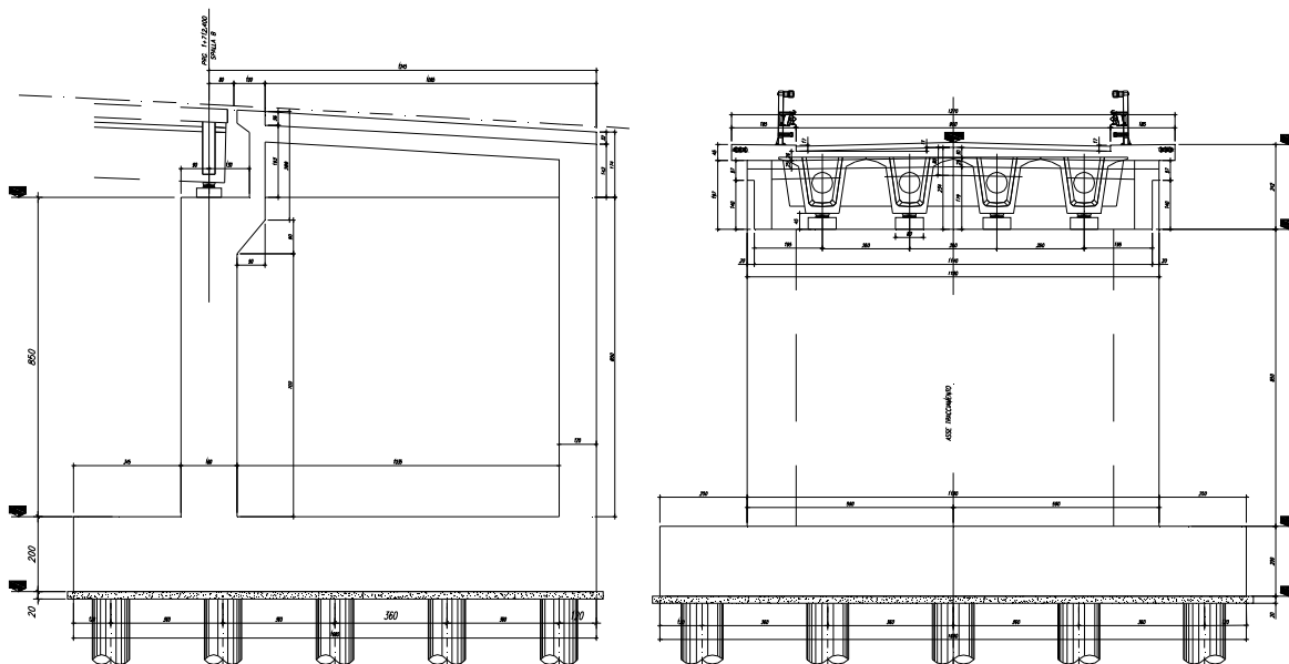
Figura 7 Carpenteria spalle 2
