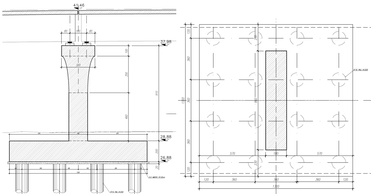
Figura 9 Sezione trasversale e Pianta delle fondazioni pile
