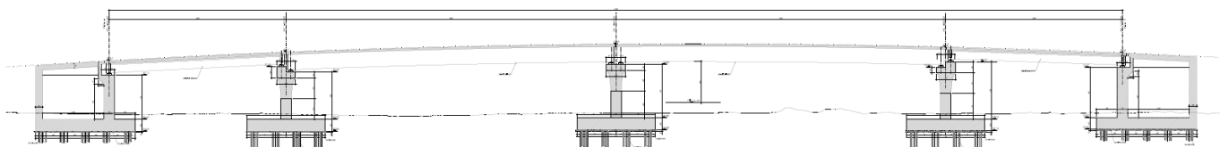
Figura 2 Sezione longitudinale
