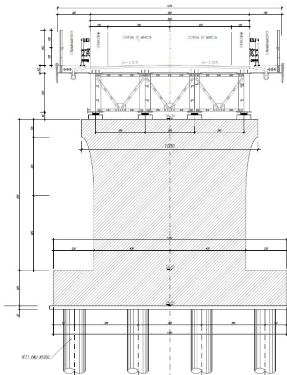
Figura 8 Sezioni longitudinali pile
