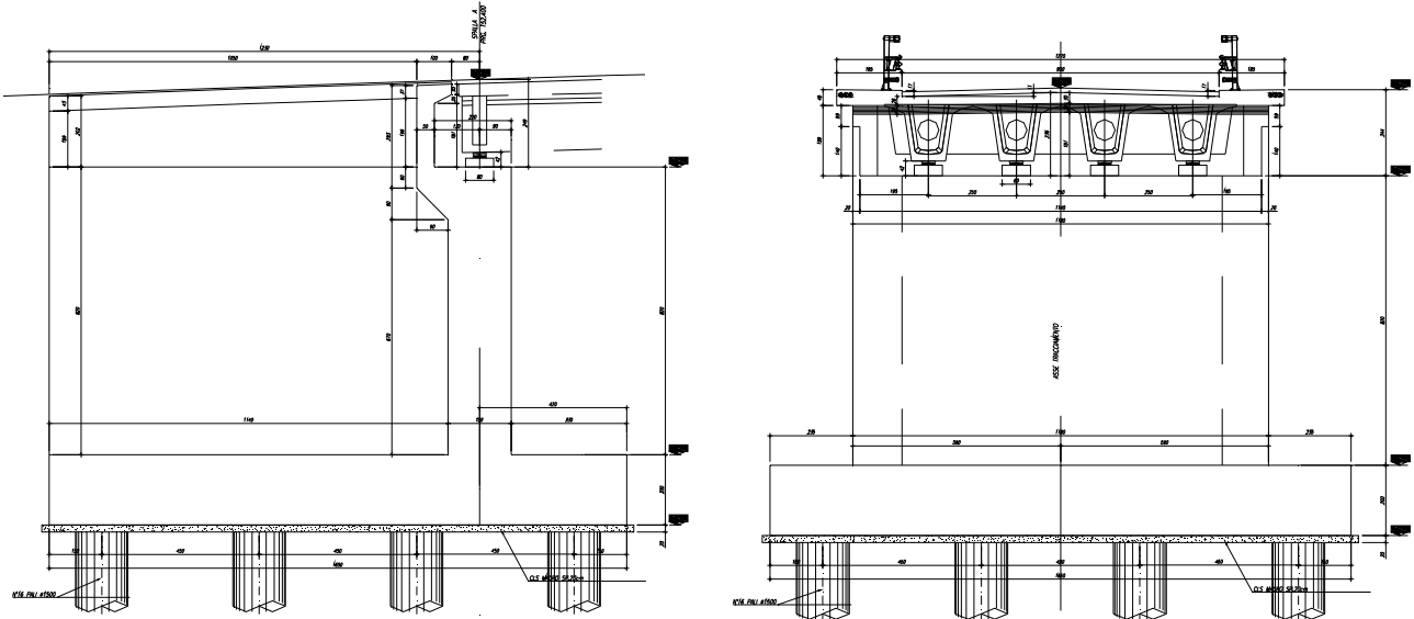
Figura 6 Carpenteria spalle 1
