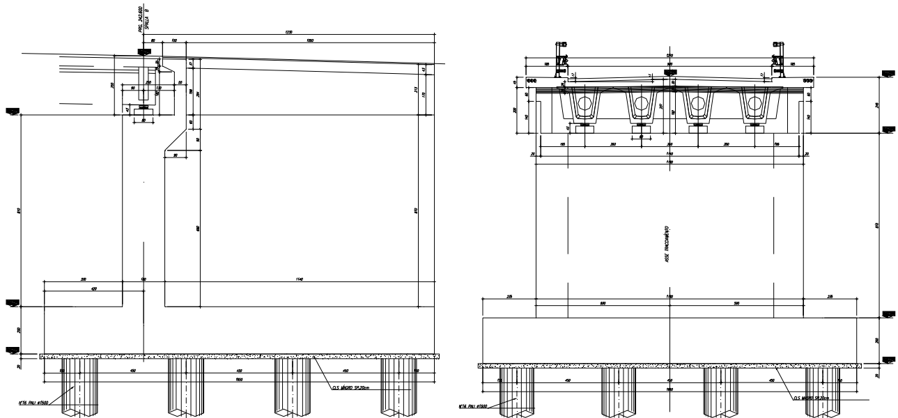
Figura 7 Carpenteria spalle 2
