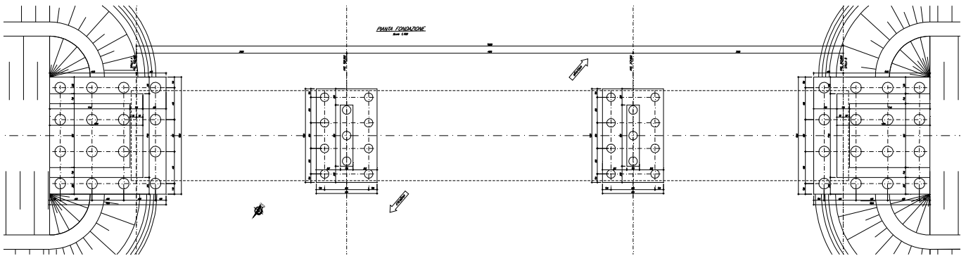
Figura 1 Pianta fondazioni
