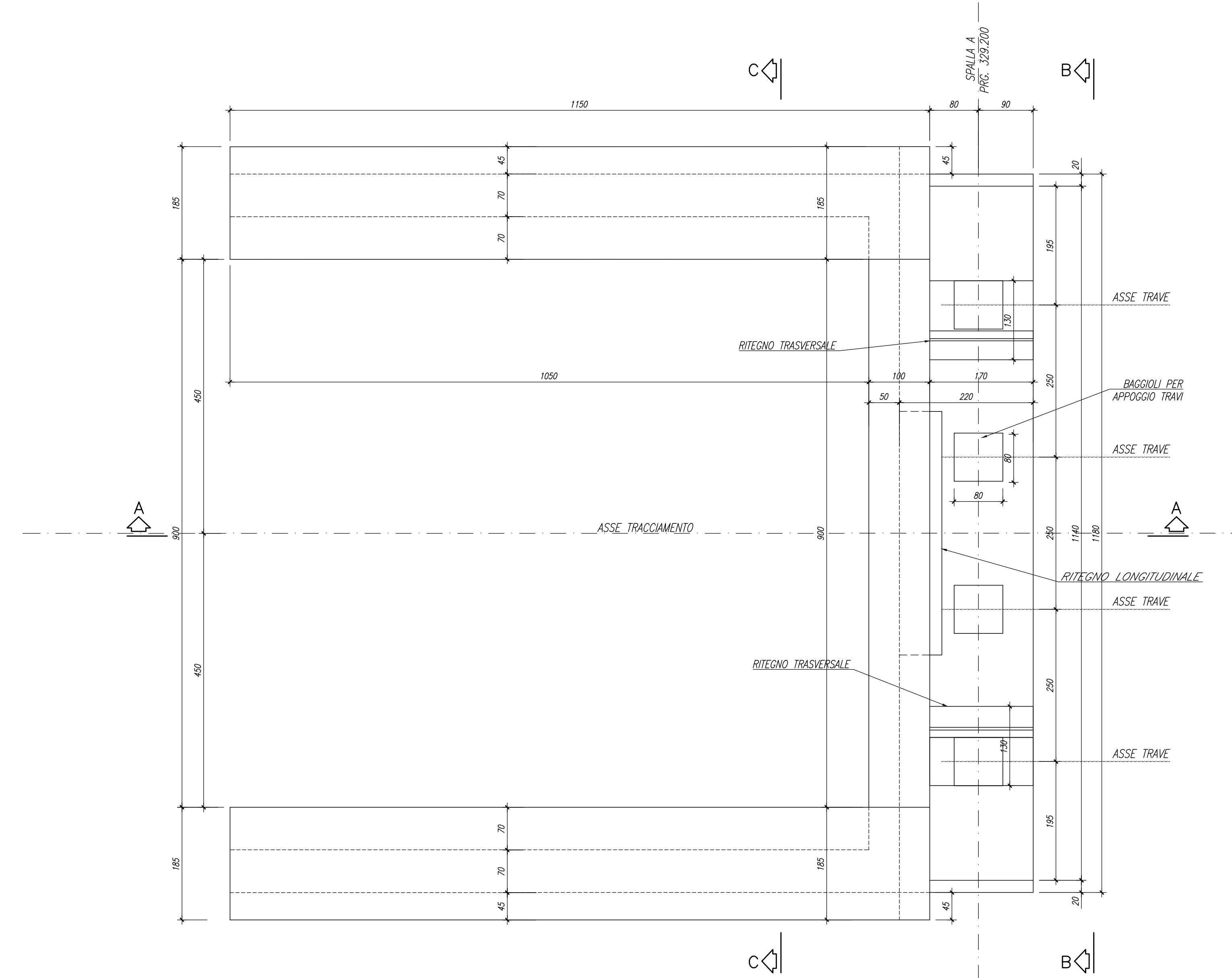
PIANTA SOMMITA' APPOGGI Scala 1:50
