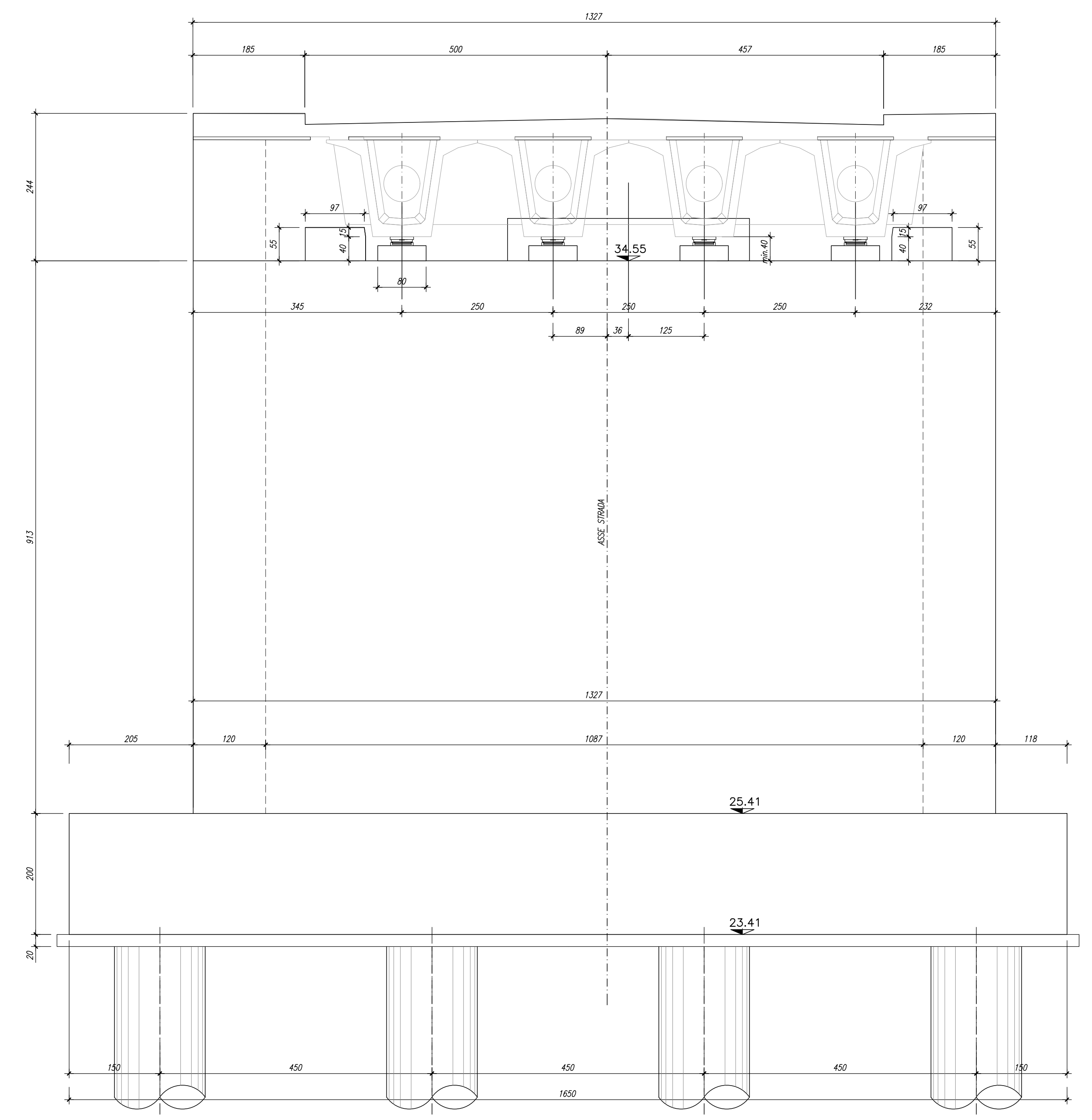
VISTA FRONTALE Scala 1:50
