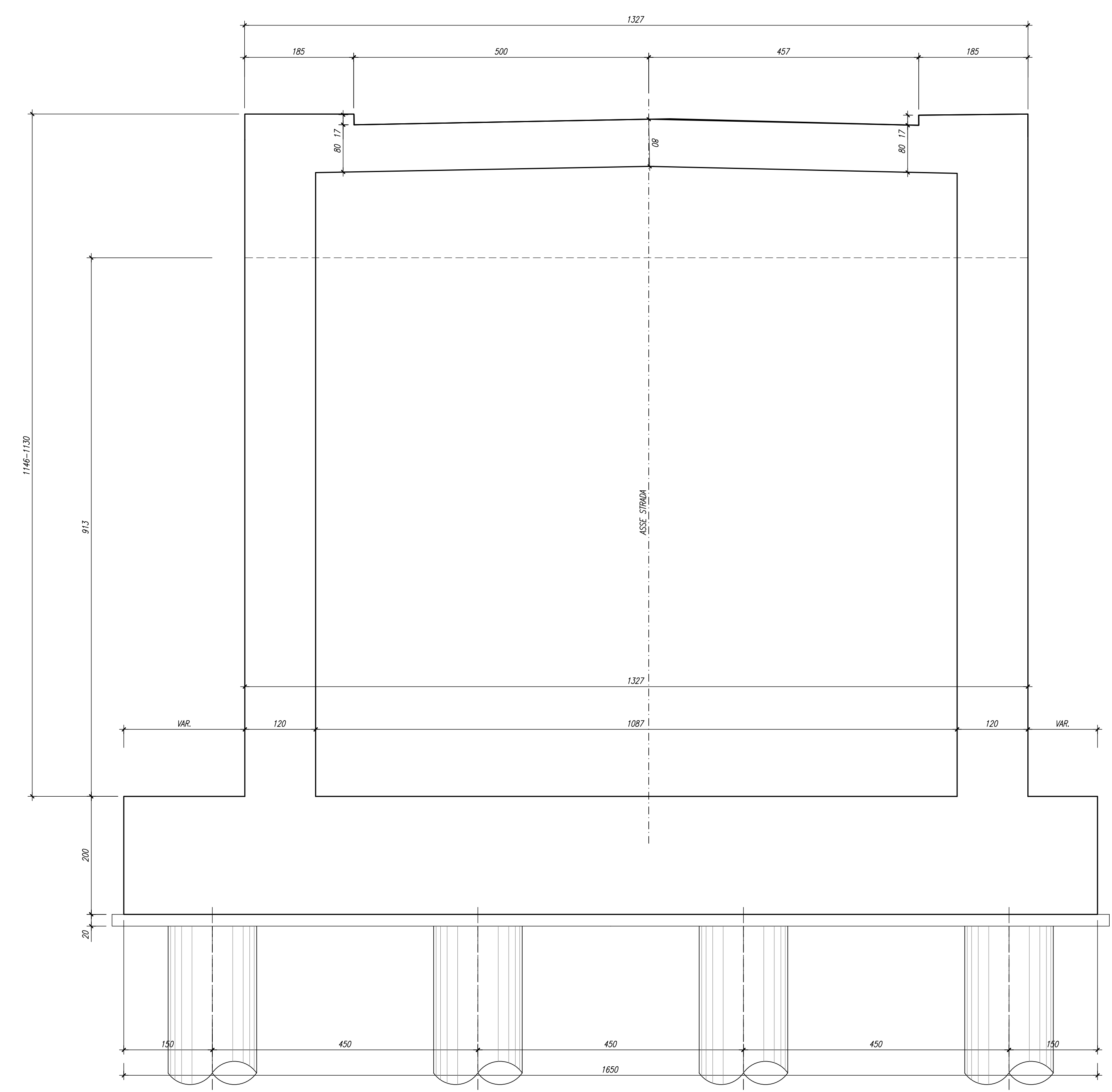
SEZIONE RISVOLTI Scala 1:50
