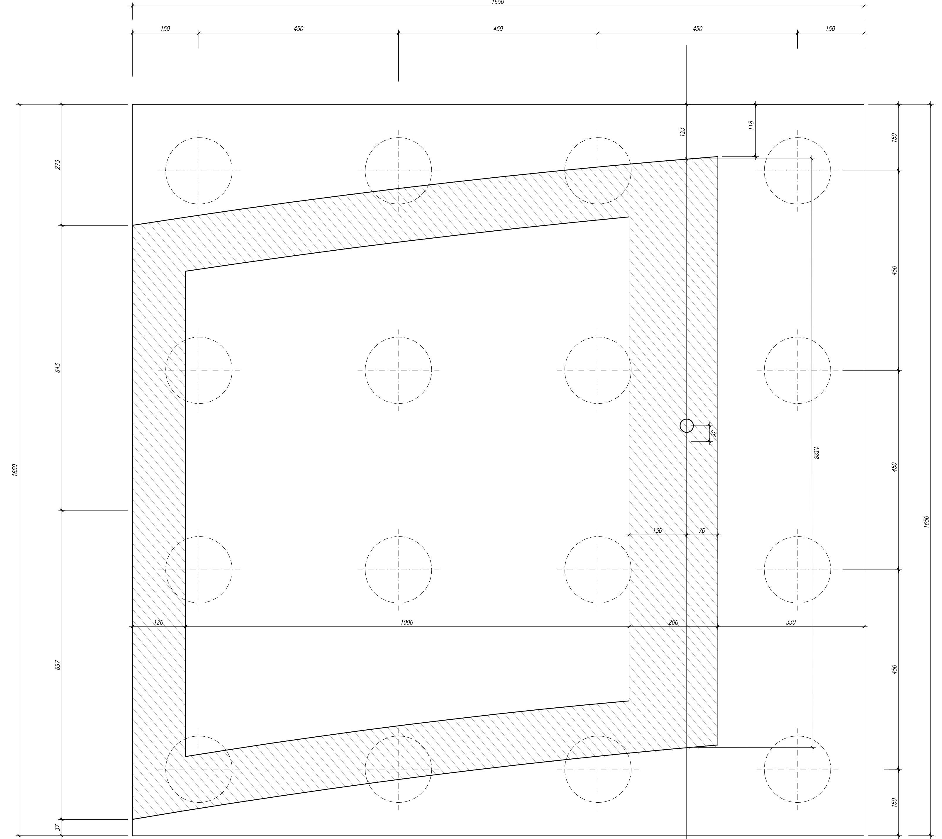
PIANTA ALLO SPICCATO Scala 1:50
