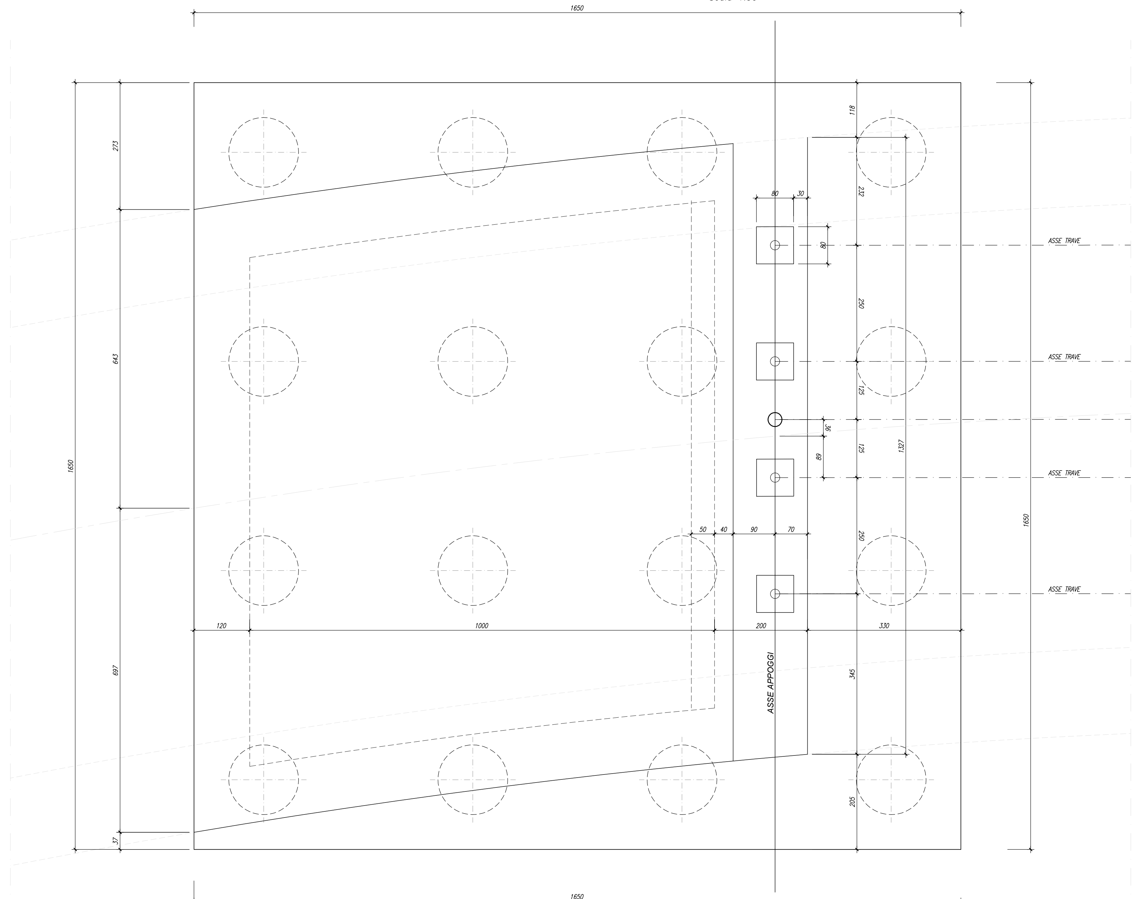
VISTA DALL'ALTO Scala 1:50
