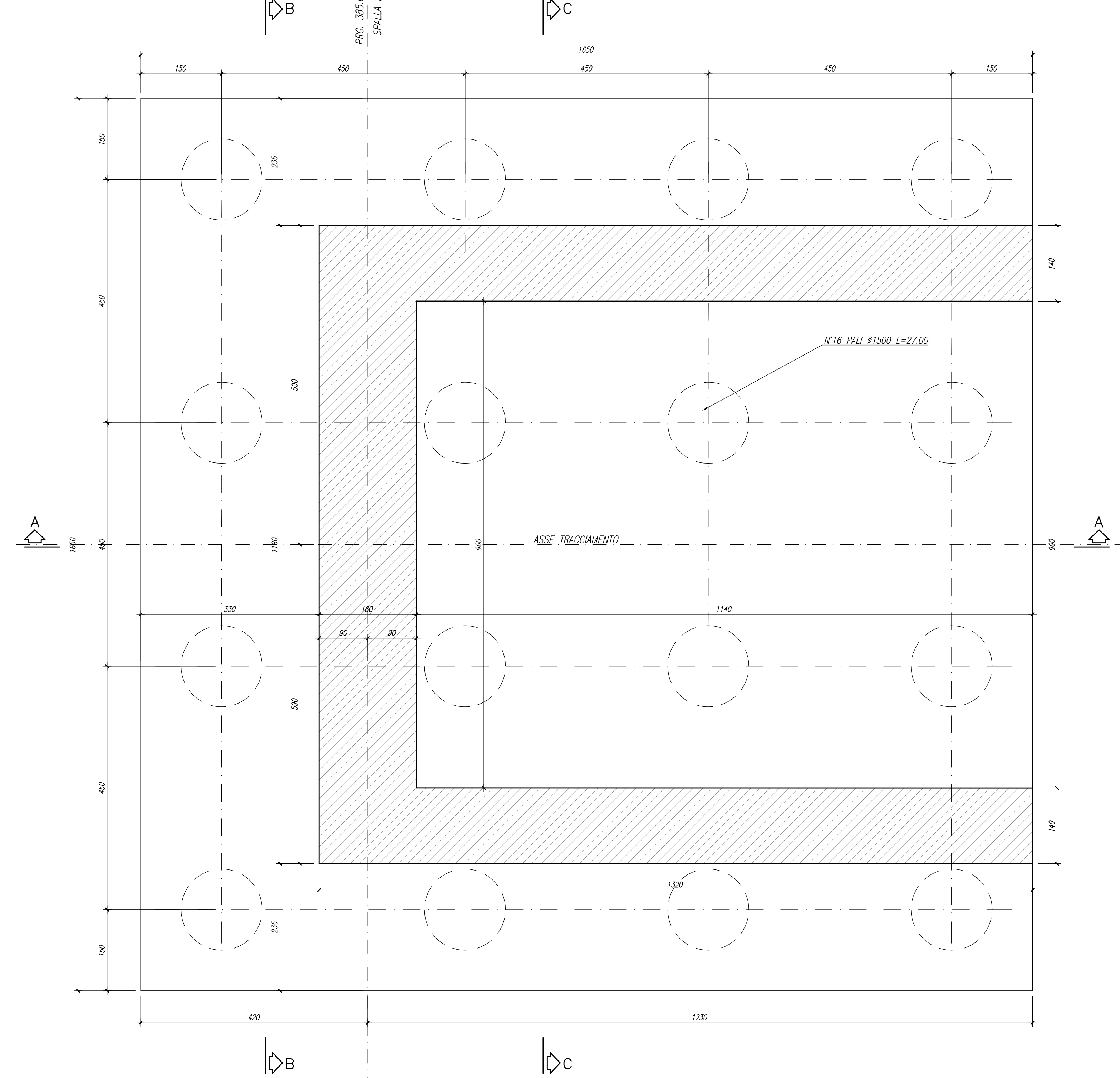
PIANTA FONDAZIONI Scala 1:50
