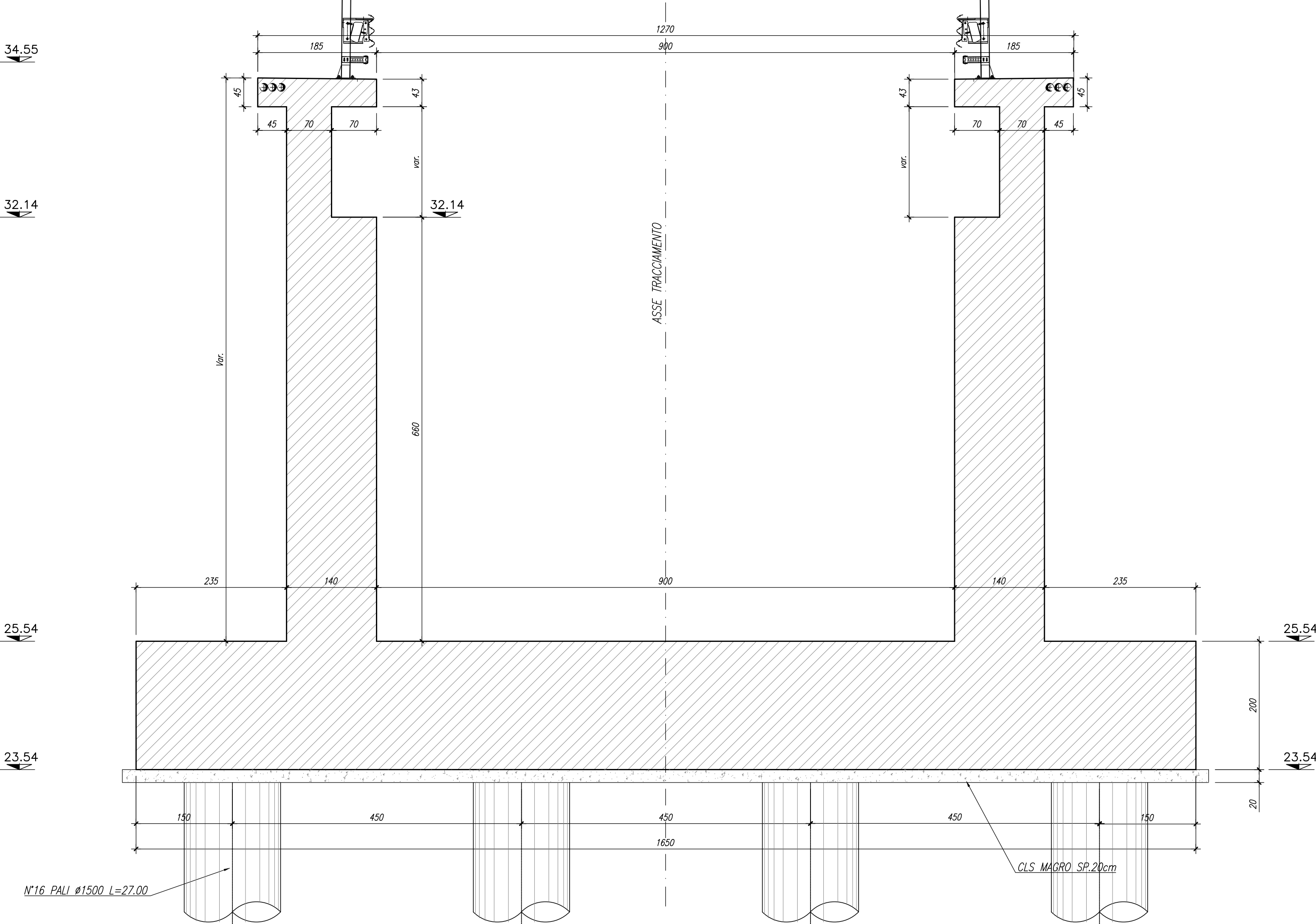
SEZIONE C-C Scala 1:50
