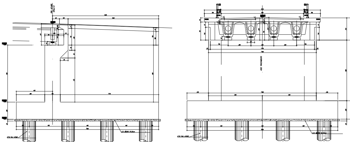
Figura 6 Carpenteria spalle 2
