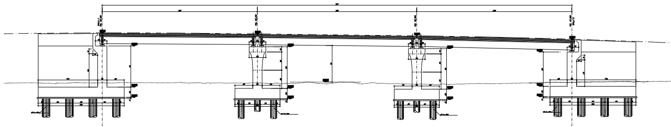
Figura 2 Profilo longitudinale
