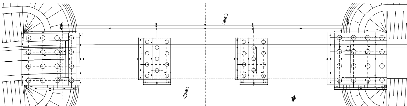
Figura 1 Pianta fondazioni
