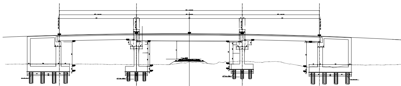
Figura 2 Profilo longitudinale
