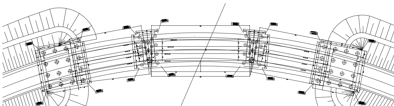
Figura 1 Pianta fondazioni
