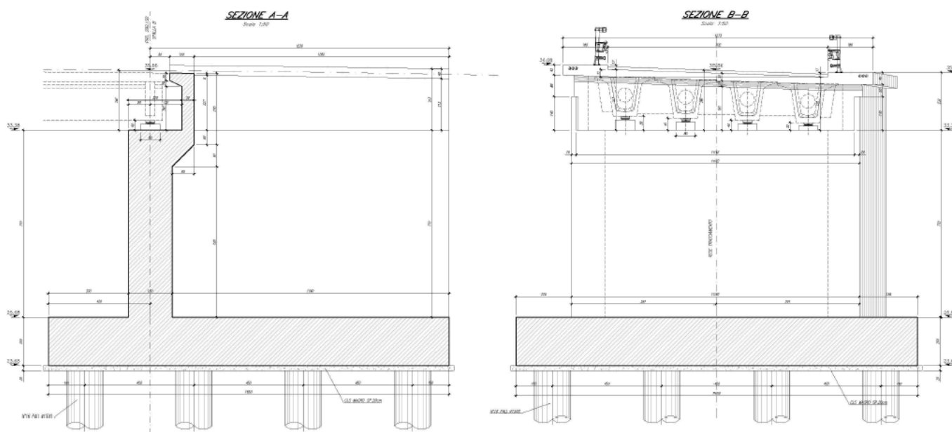
Figura 7 Carpenteria spalle 2
