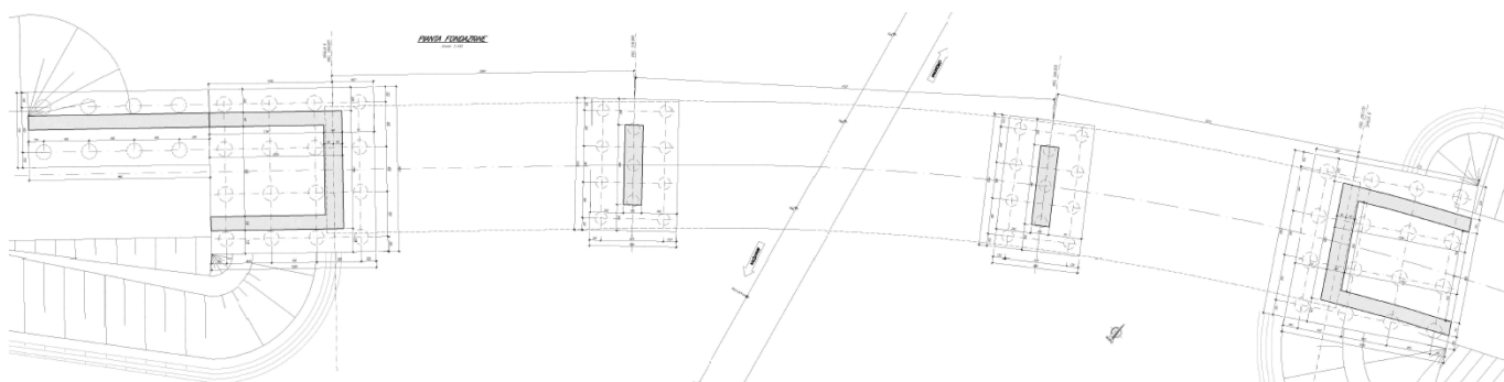
Figura 1 Pianta fondazioni
