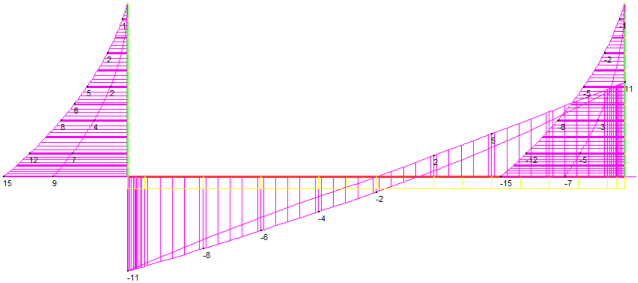
Figura 17 Involupto SLE: sollecitazioni taglianti
