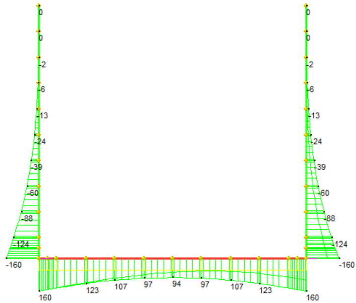
Figura 4 Involupto SLE: Momenti flettenti
