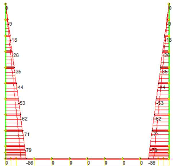
Figura 3 Involuppo SLU/Sisma: sforzo normale
