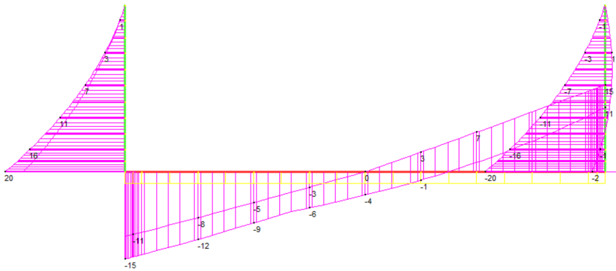
Figura 14 Involuppo SLU/Sisma: sollecitazioni taglianti
