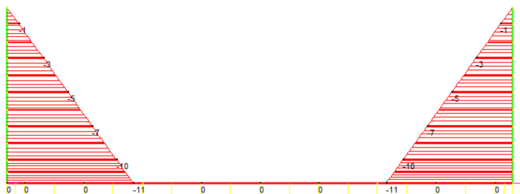
Figura 18 Involucro SLE: sforzo normale
