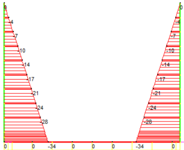
Figura 12 Involuppo SLE: sforzo normale
