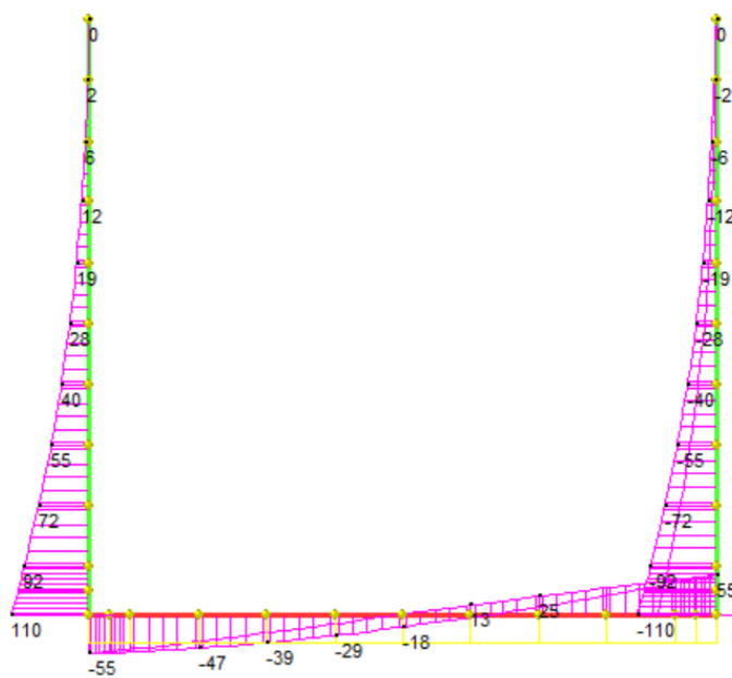
Figura 5 Involupto SLE: sollecitazioni taglianti
