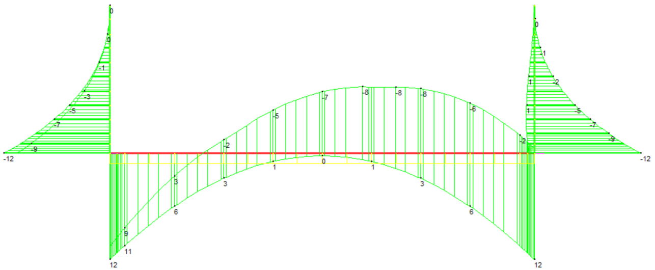
Figura 13 Involuppo SLU/Sisma: Momenti flettenti
