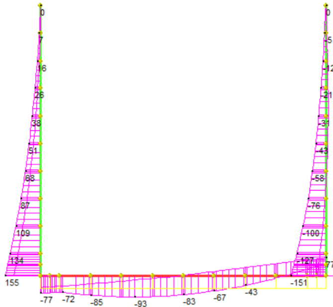
Figura 2 Involuppo SLU/Sisma: sollecitazioni taglianti
