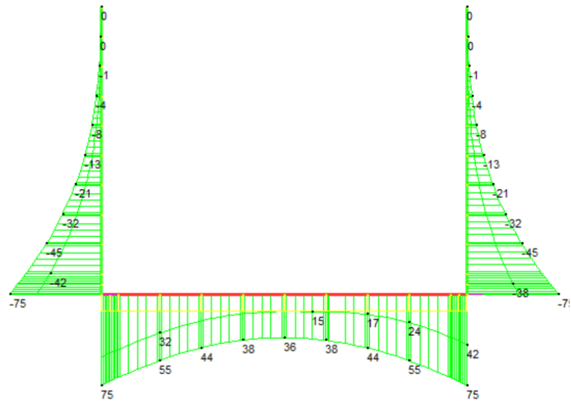
Figura 10 Inviluppo SLE: Momenti flettenti
