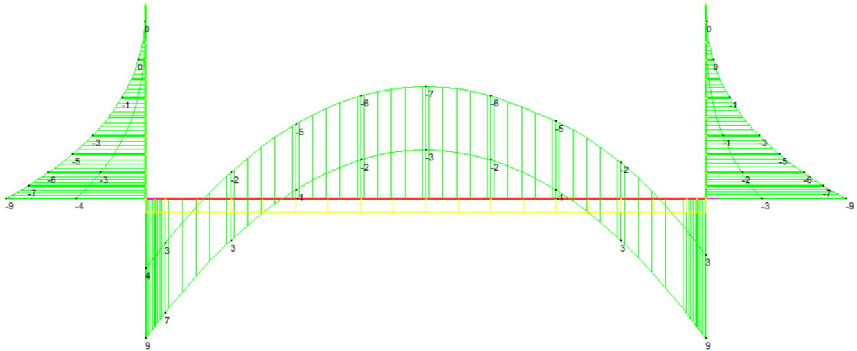
Figura 16 Involupto SLE: Momenti flettenti
