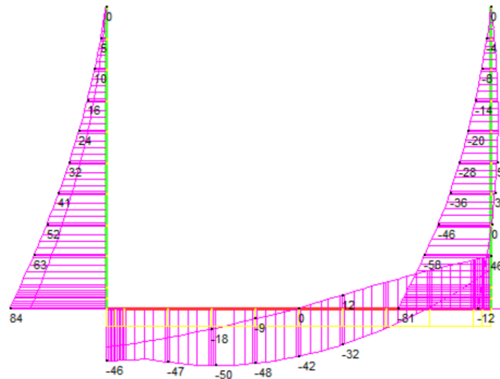
Figura 8 Involuppo SLU/Sisma: sollecitazioni taglianti
