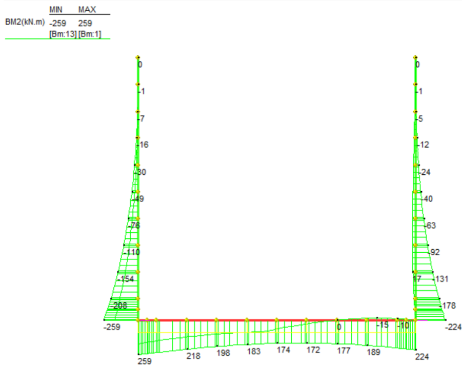
Figura 1 Involuppo SLU/Sisma: Momenti flettenti
