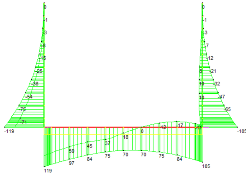
Figura 7 Involuppo SLU/Sisma: Momenti flettenti
