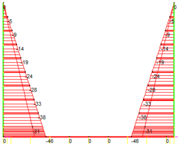
Figura 9 Involuppo SLU/Sisma: sforzo normale
