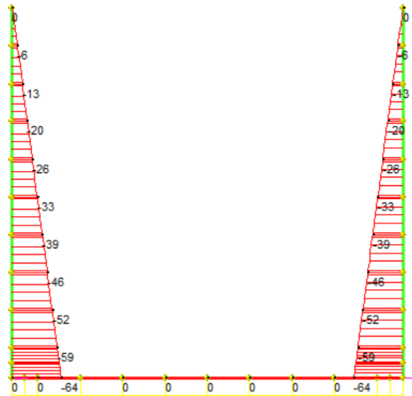
Figura 6 Involuppo SLE: sforzo normale
