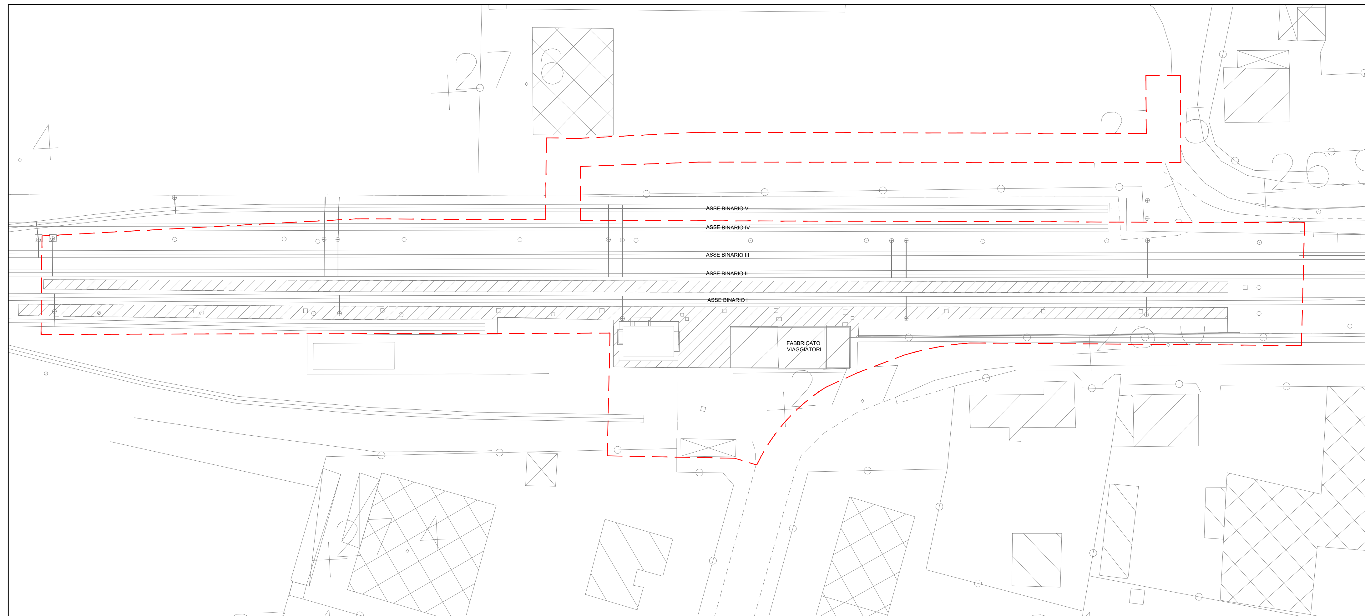
1 PLANIMETRIA ANTE OPERAM scala 1:500
