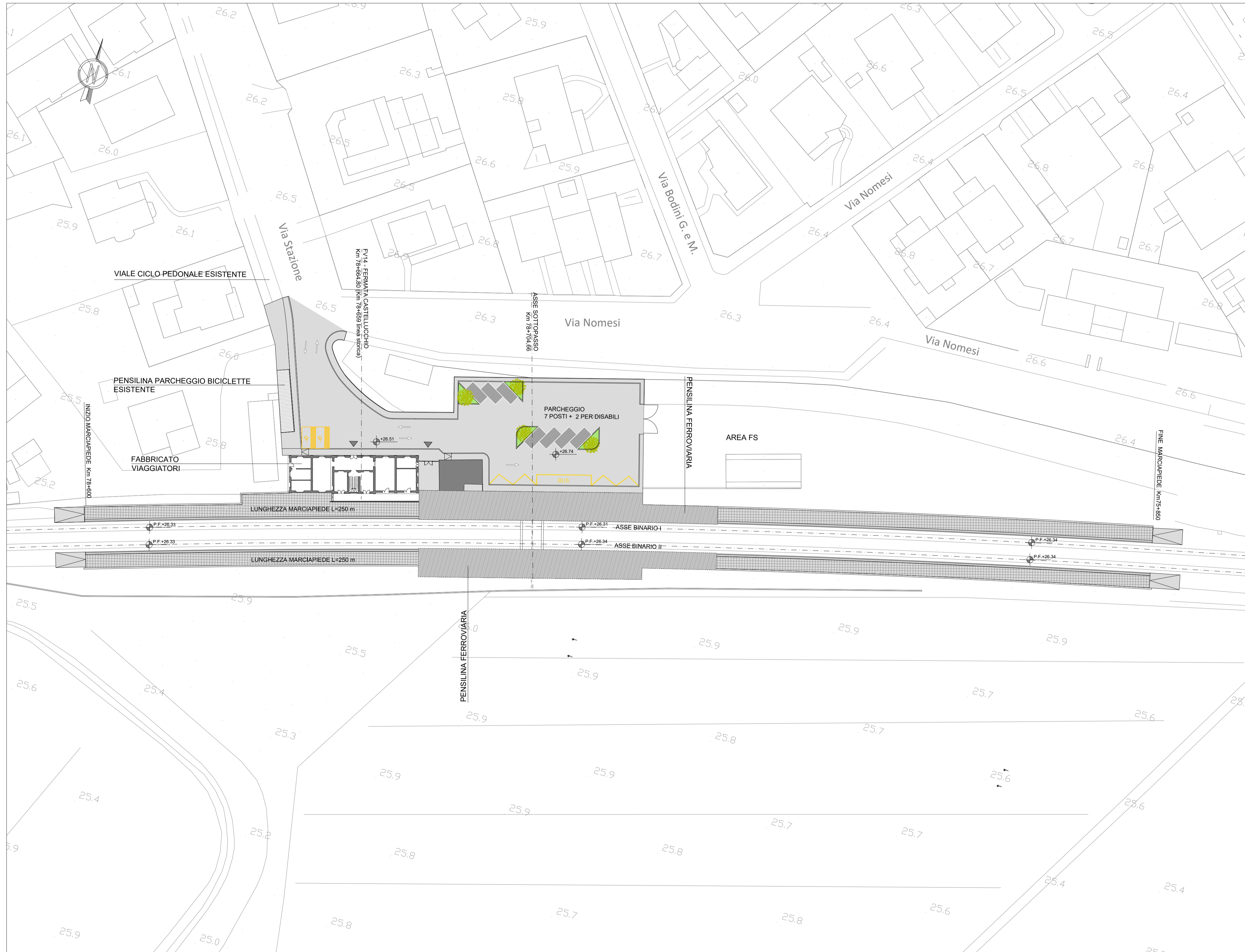
1 PLANIMETRIA GENERALE scala 1:500
