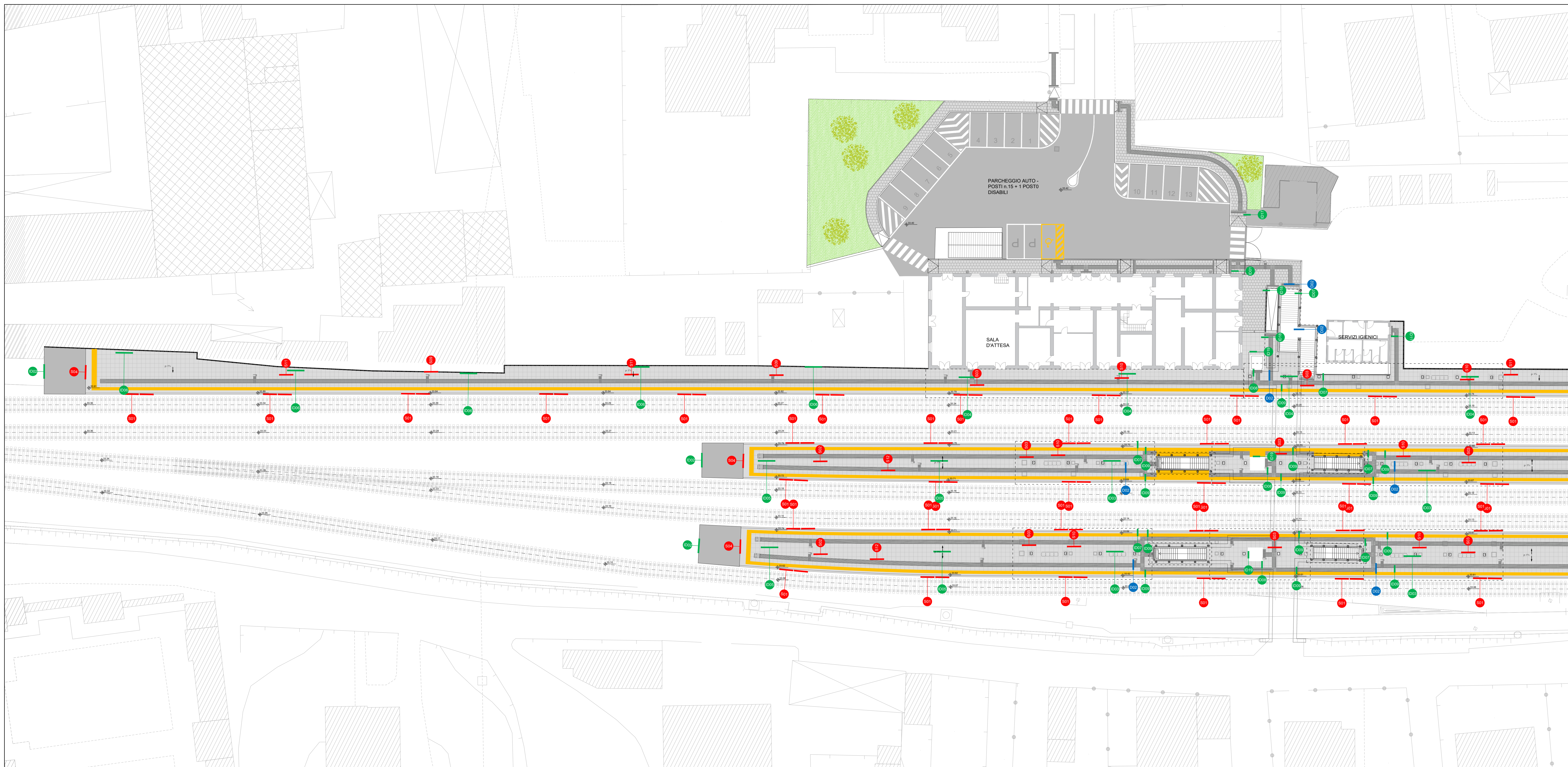
1 PIANTA QUOTA BANCHINA STRALCIO 1 scala 1:200
