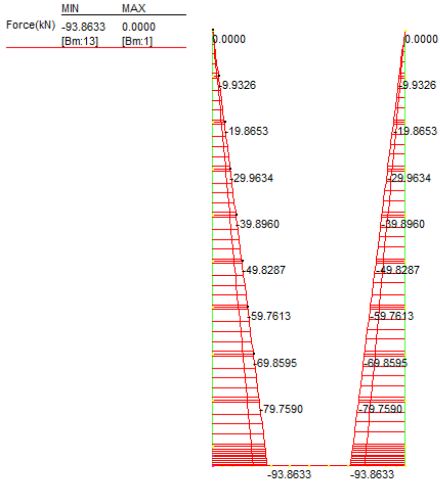
Figura 3 Involuppo SLU/Sisma: sforzo normale
