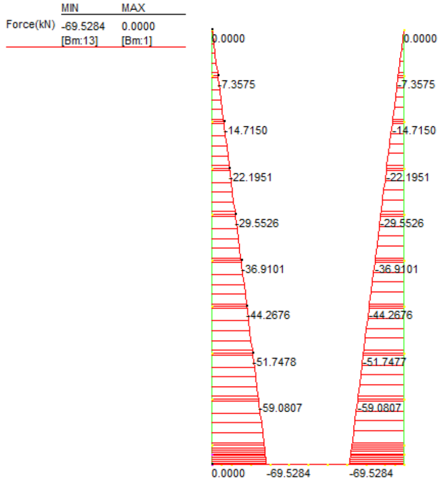
Figura 6 Involuppo SLE: sforzo normale
