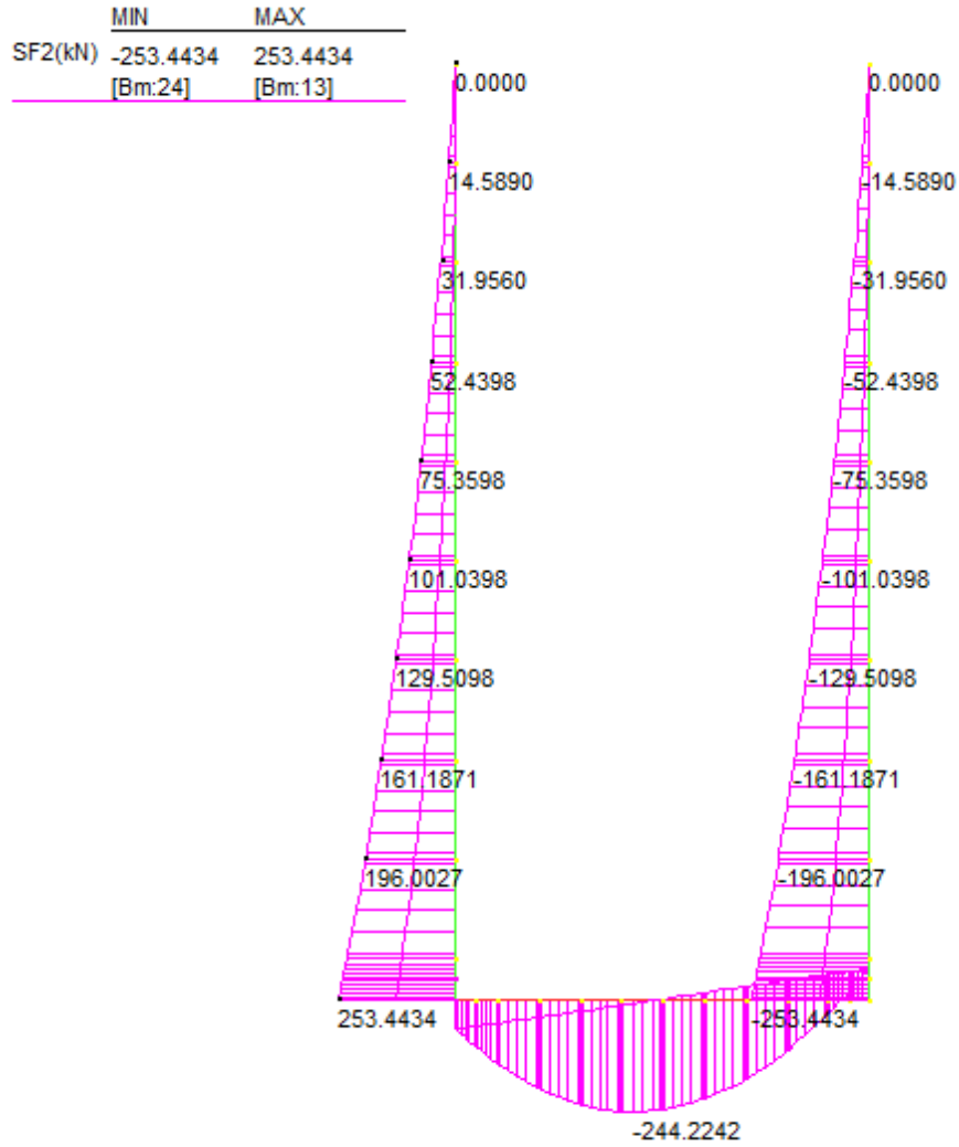
Figura 5 Involuppo SLE: sollecitazioni taglianti
