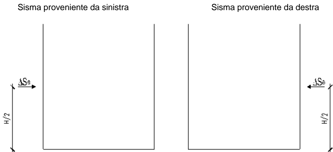
Figura 8 Spinta sismica del terreno secondo la teoria di Wood
