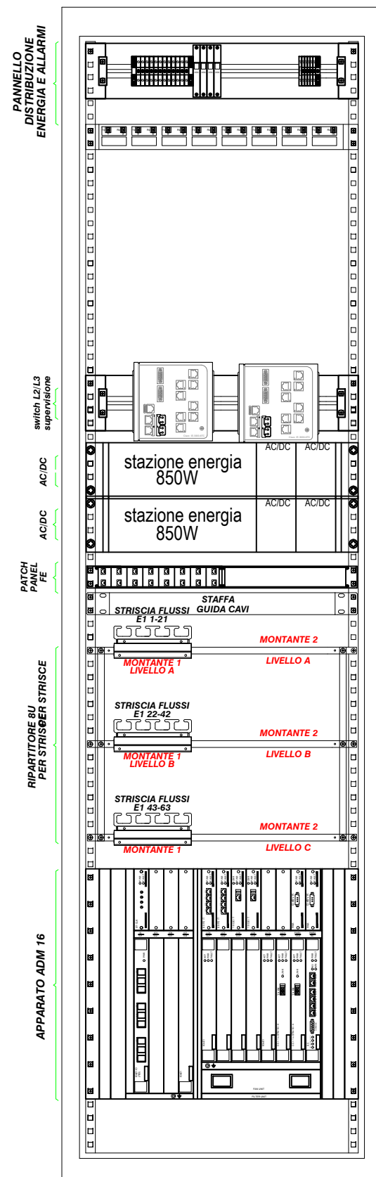
Telaio N3 di installazione ADM 16 600X300X2200 mm
