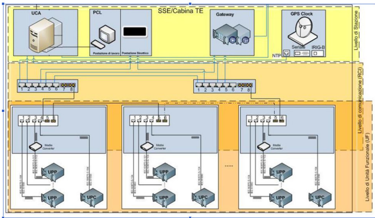
Figura 2 Architettura fisica del SDG
