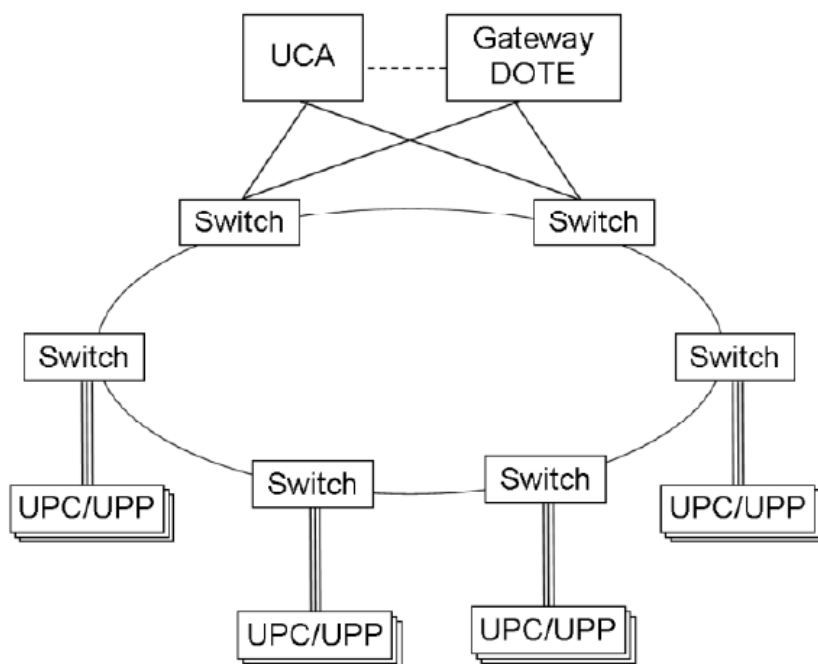
Figura 4 Architettura di rete di comunicazione ad anello
