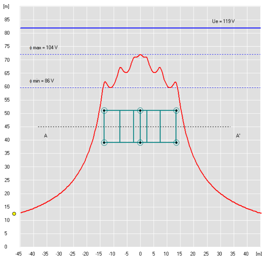
Figura 4 - Potenziale della maglia longitudinale
