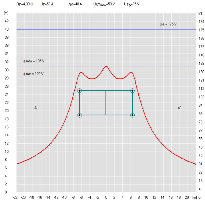
Figura 9 - Potenziale della maglia longitudinale
