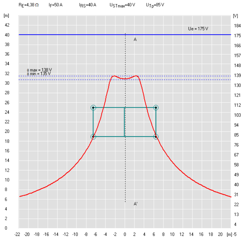
Figura 10 - Potenziale della maglia trasversale
