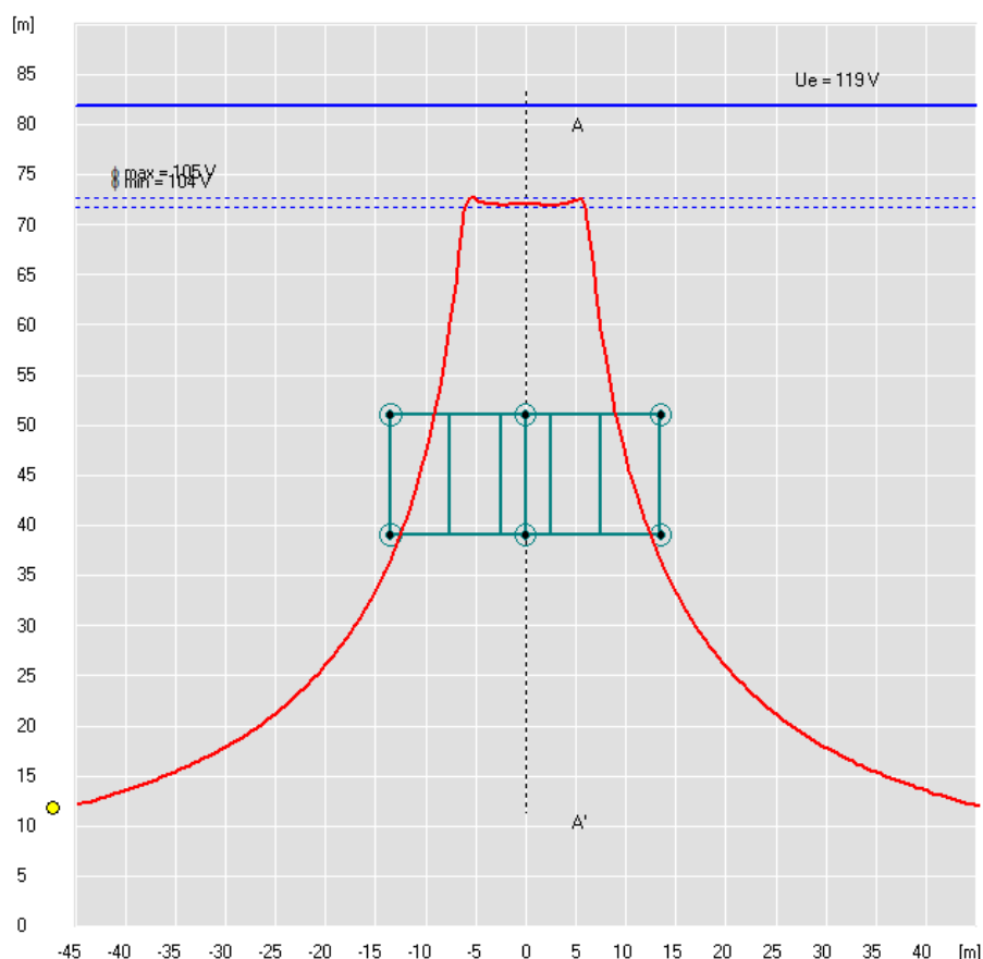
Figura 5 - Potenziale della maglia trasversale
