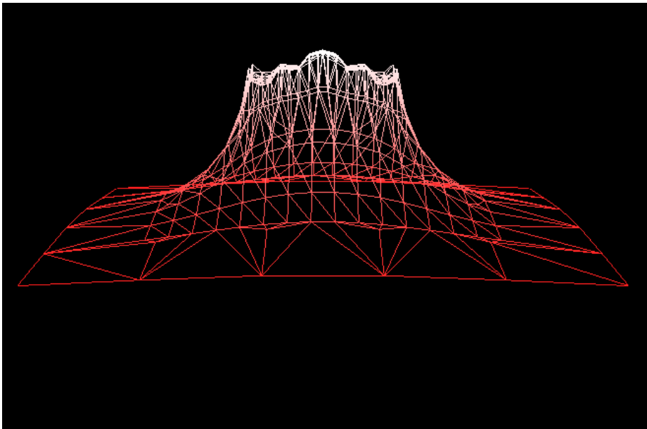
Figura 3 - Potenziale della maglia in 3D
