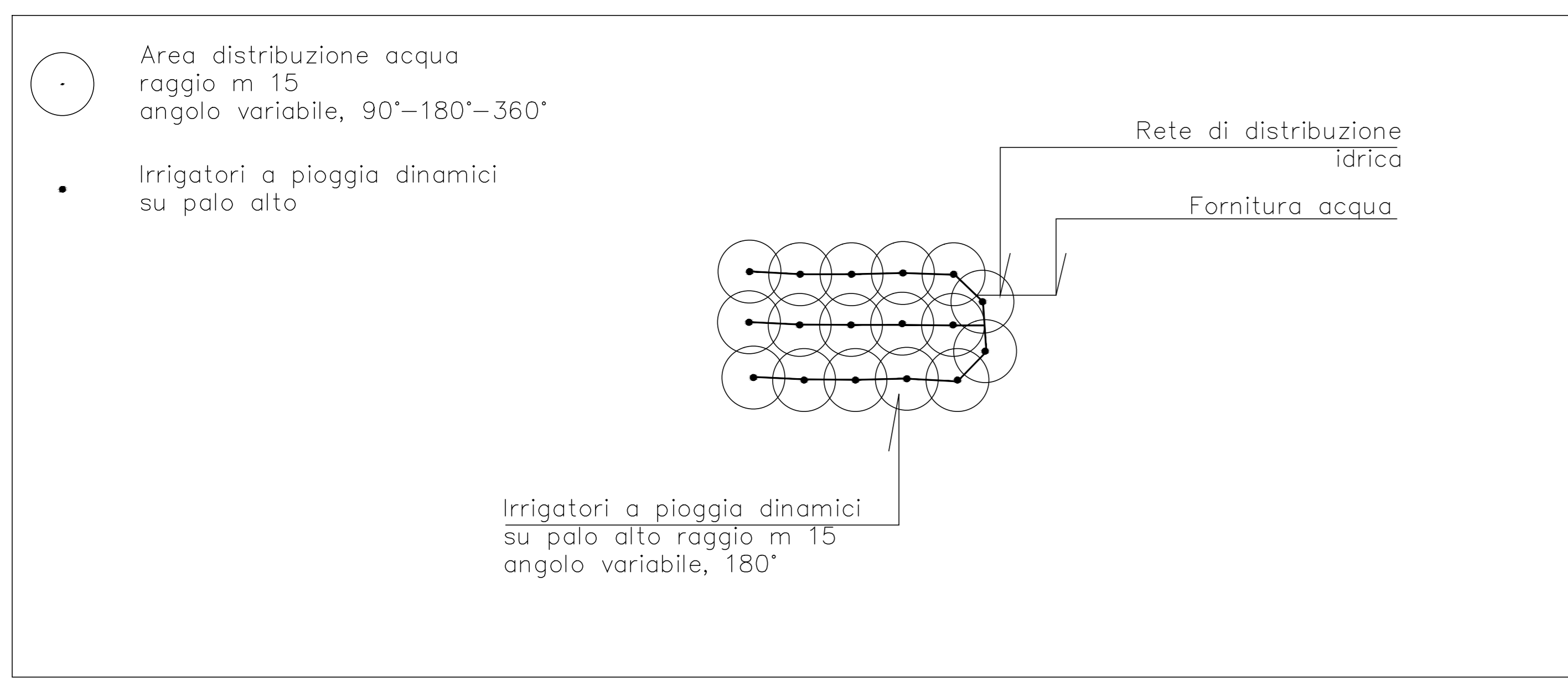
2) Schema impianto d'irrigazione Scala 1:2000
