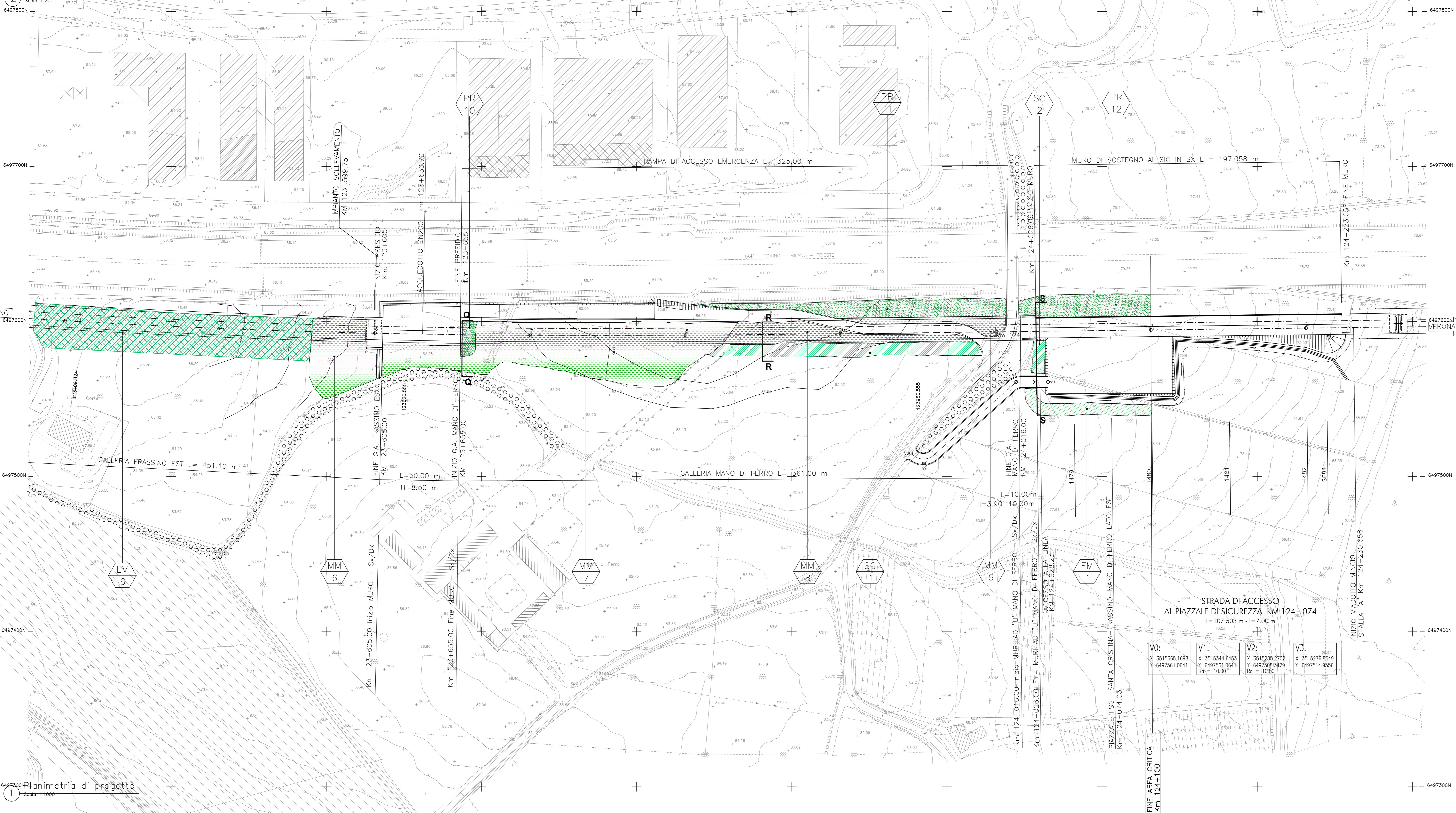
2 Schema di impianto d'irrigazione: planimetria
