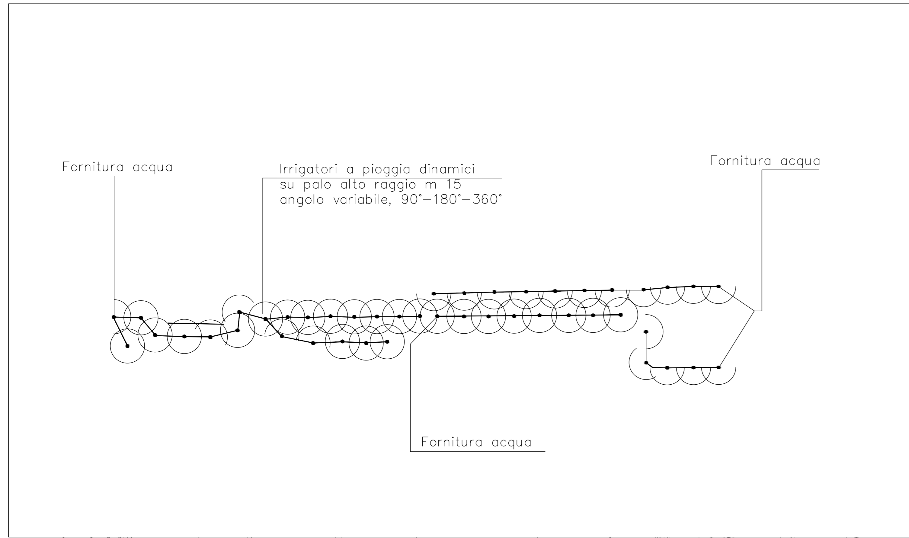
2 Schema di impianto d'irrigazione: planimetria
