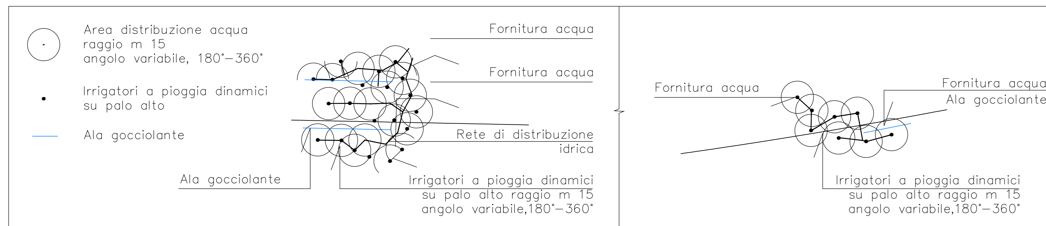
2 Schema d'impianto d'irrigazione: planimetria Scala 1:2000
