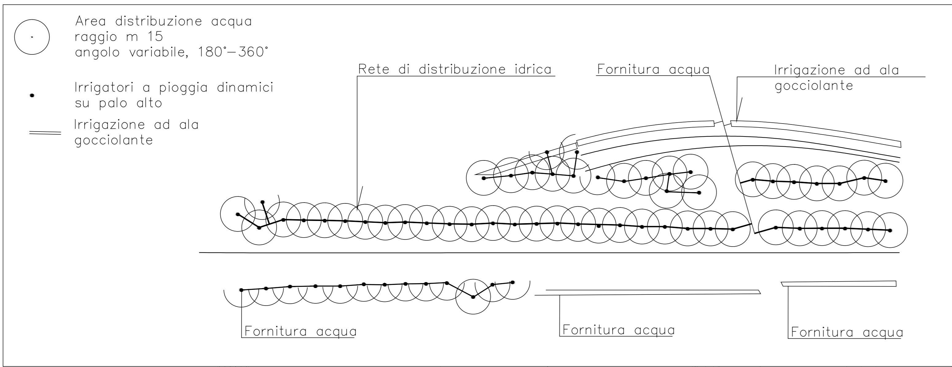
2) Schema di impianto d'irrigazione: planimetria Scala 1:2000
