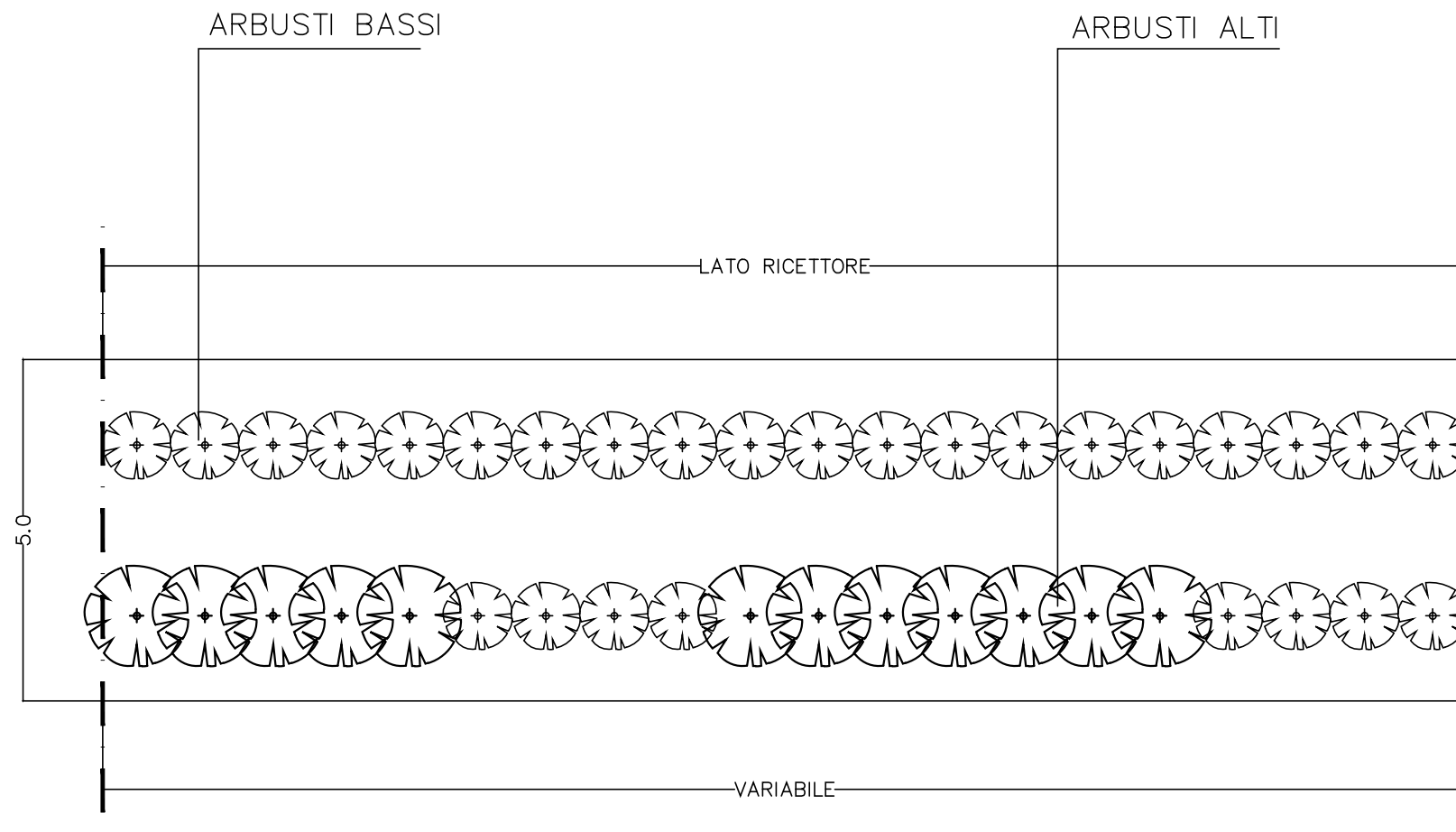
1 Schema planimetrico Scala 1:100
