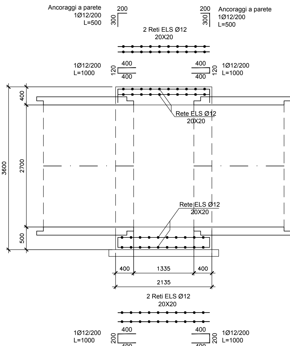
SEZIONE B-B
