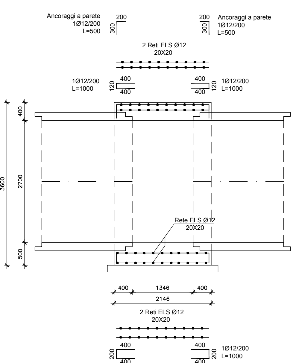
SEZIONE B-B
