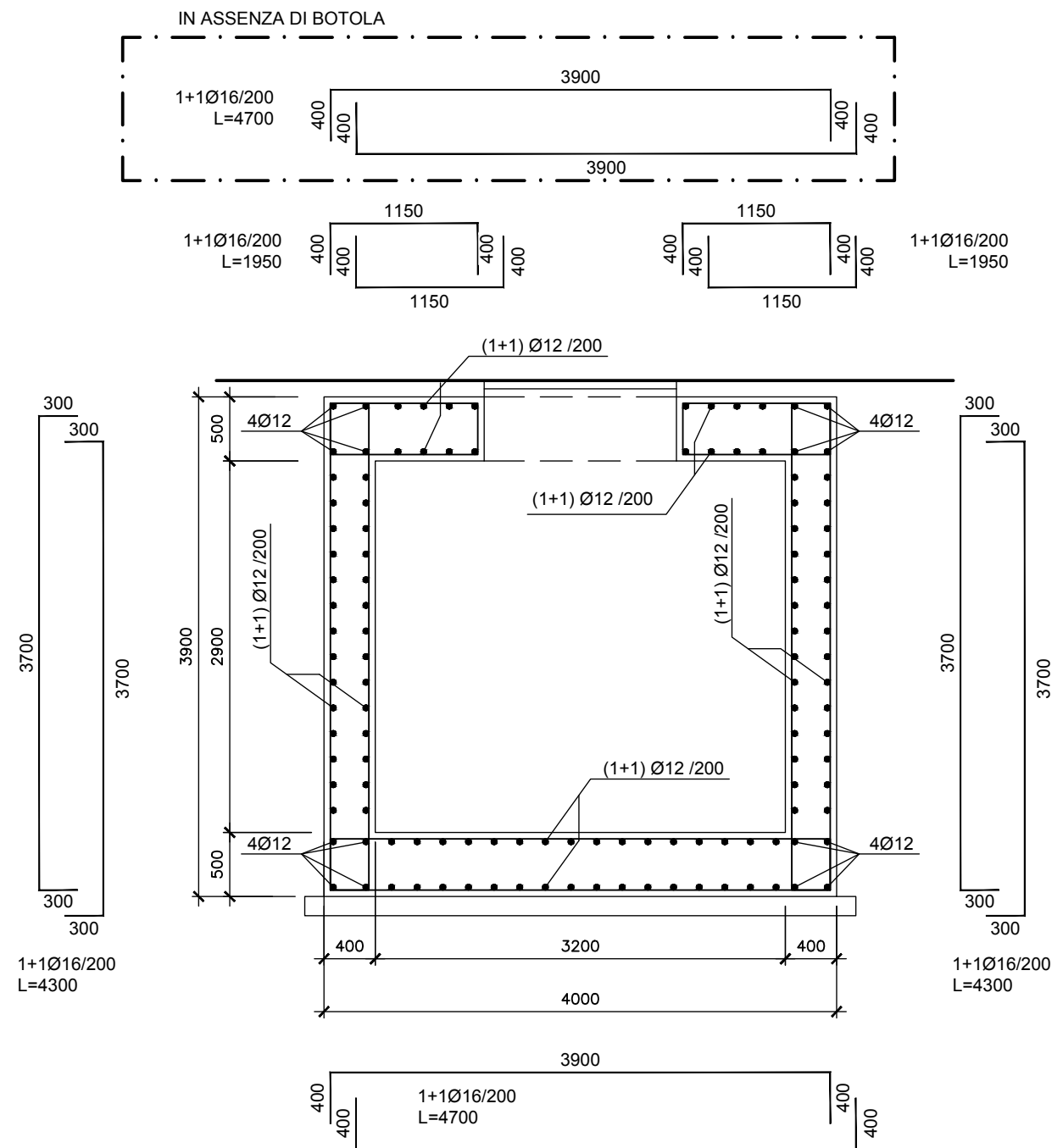
SEZIONE B-B
