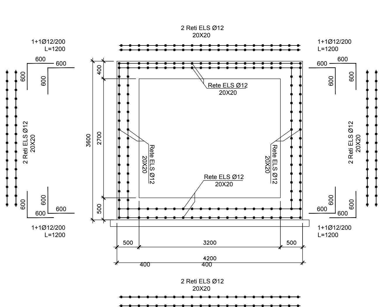
SEZIONE A-A
