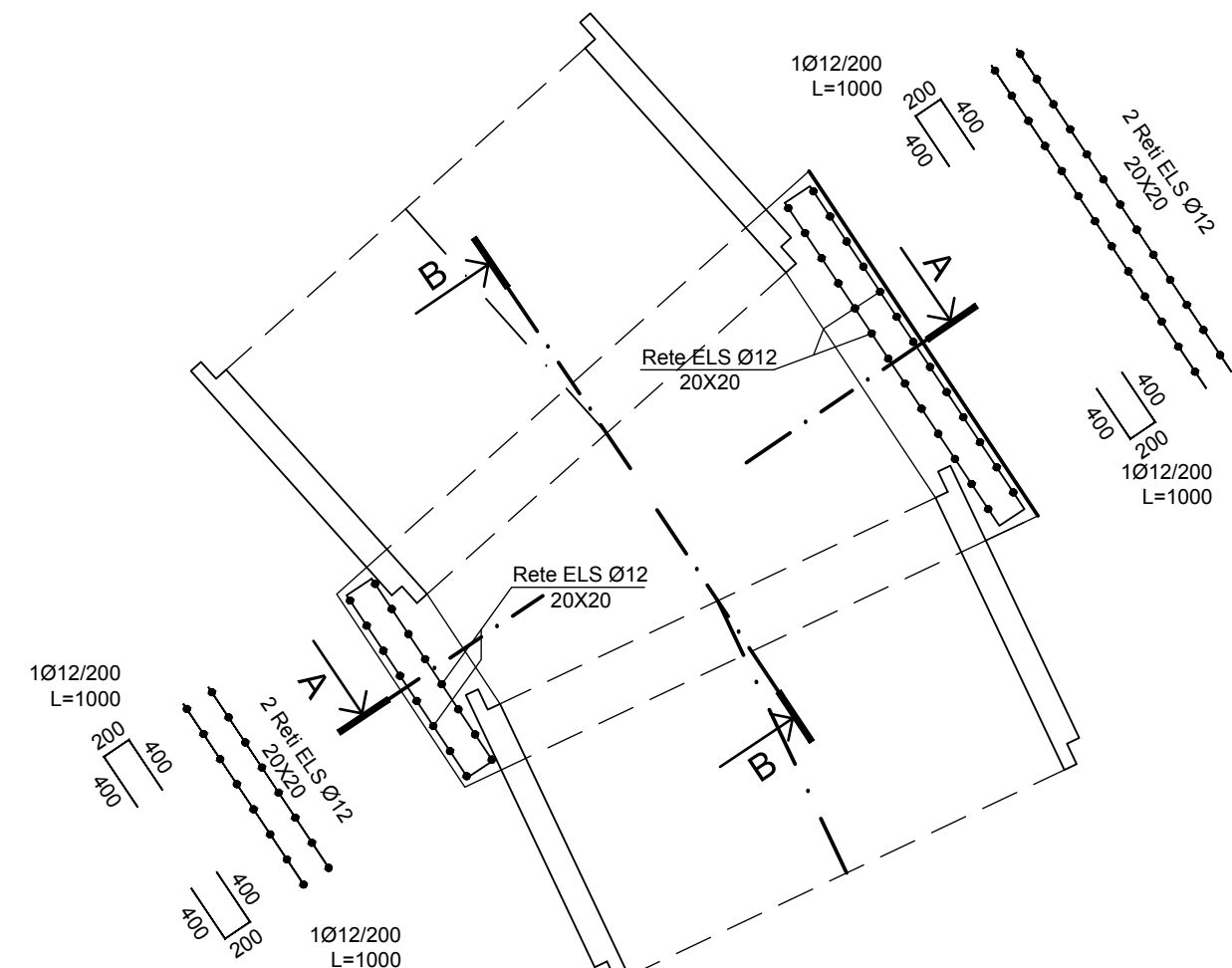
PIANTA
