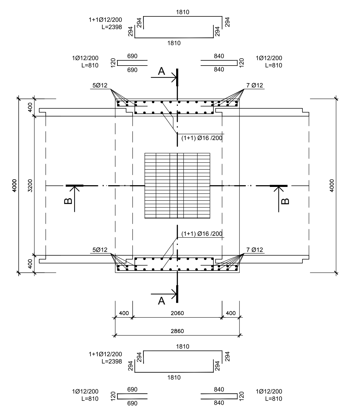
PIANTA
