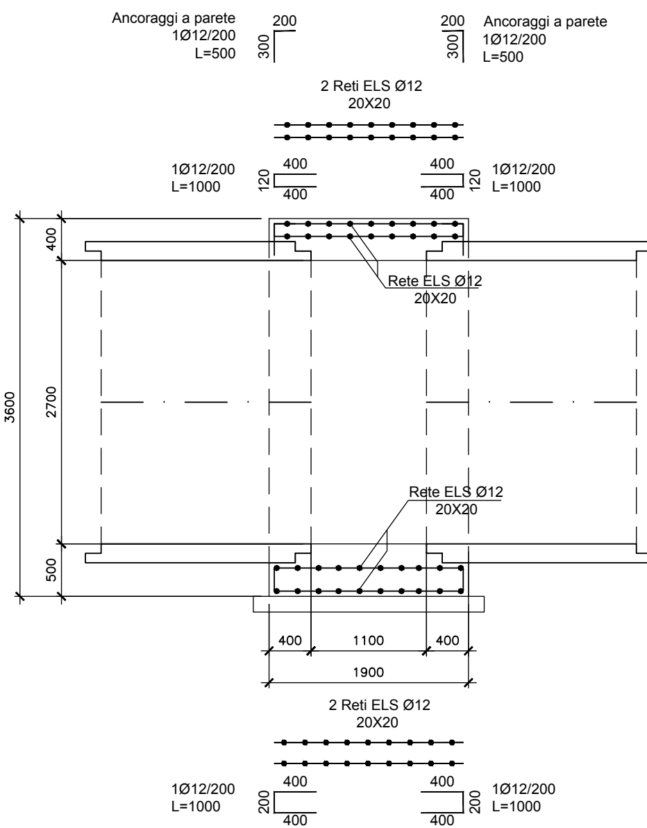
SEZIONE B-B
