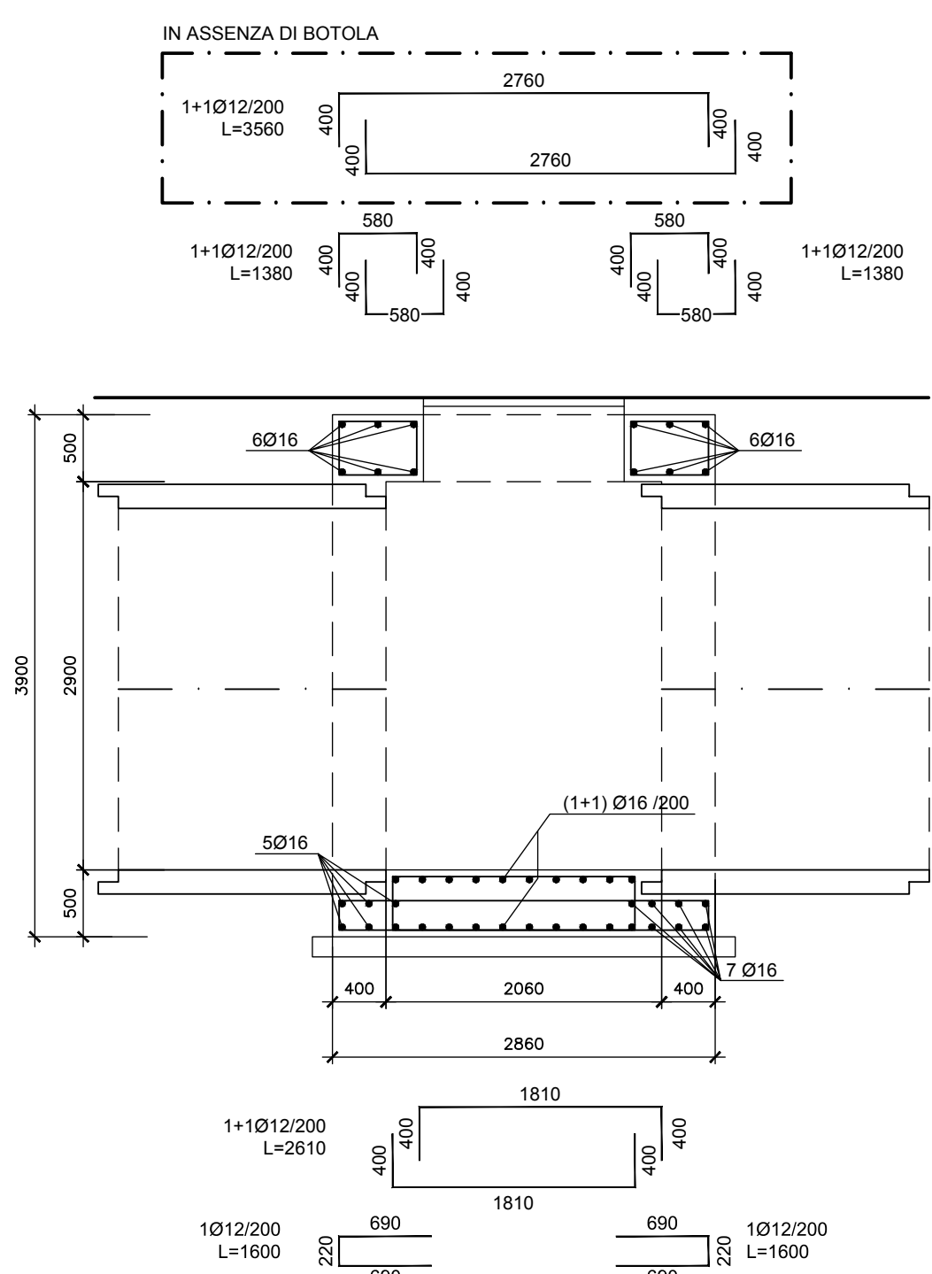
PIANTA
