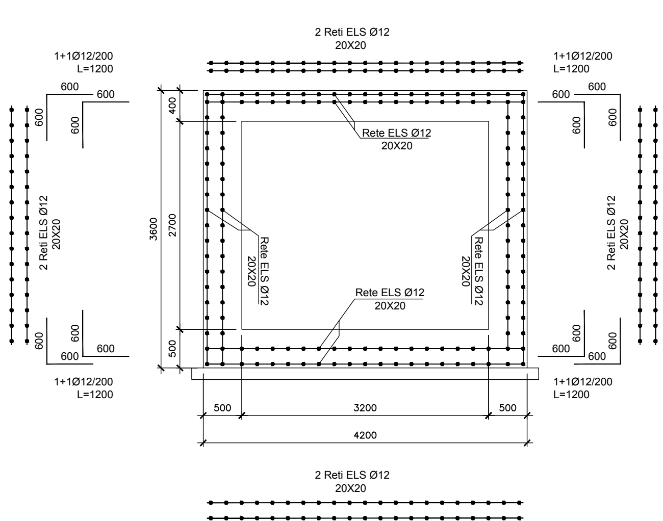
SEZIONE A-A
