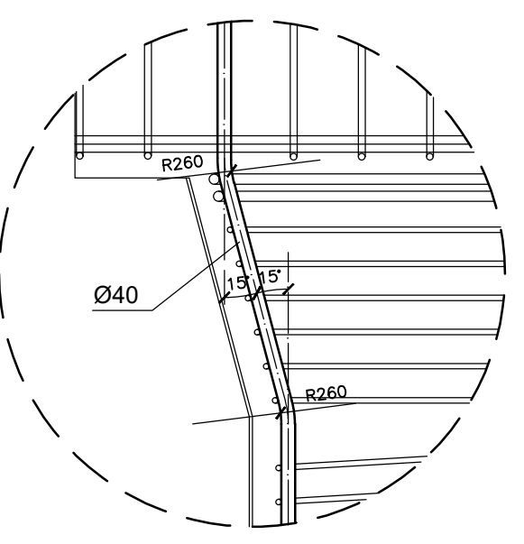
DETTAGLIO 1 Scala 1:20
