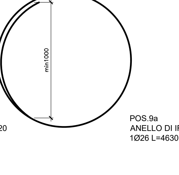
SEZIONE G-G Scala 1:20
