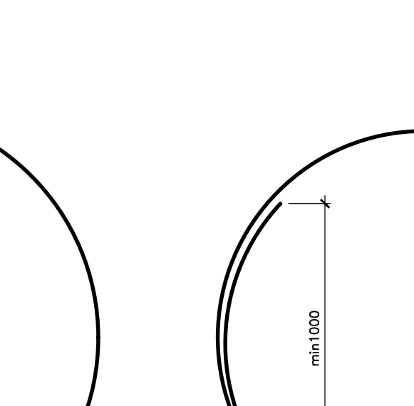
SEZIONE C-C Scala 1:20
