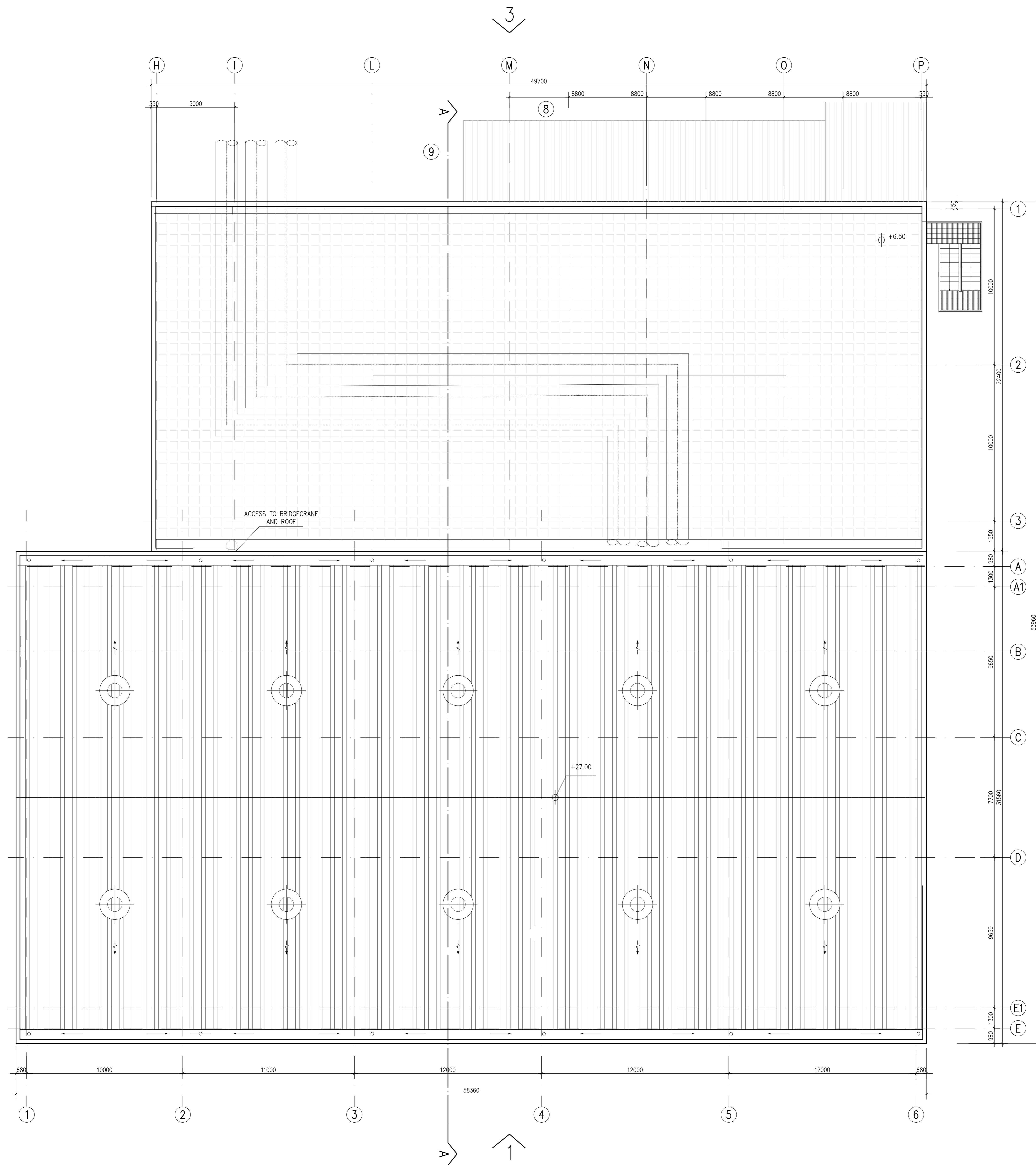
PIANTA COPERTURA SCALE 1:100
