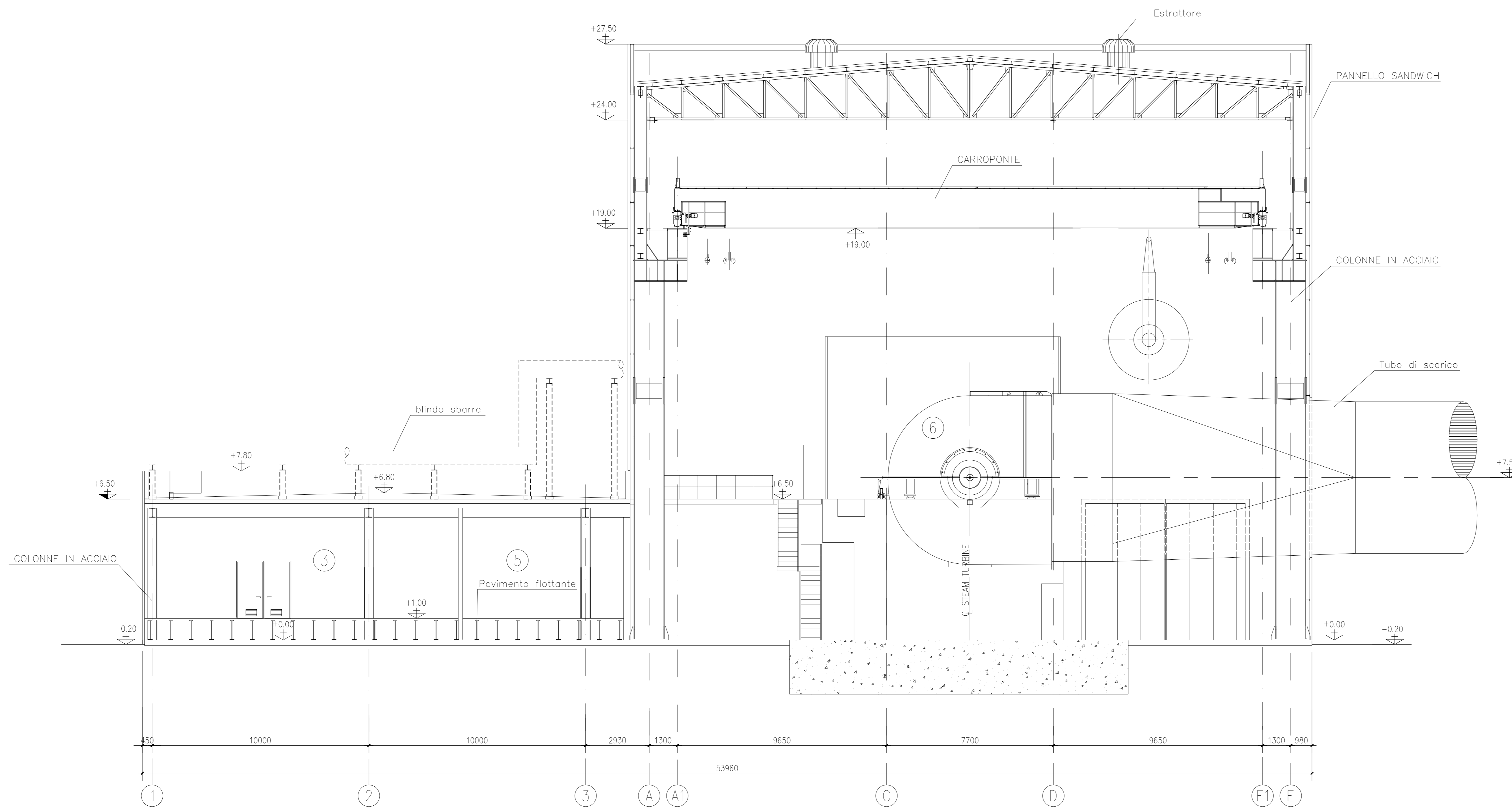
SEZIONE A-A SCALE 1:100
