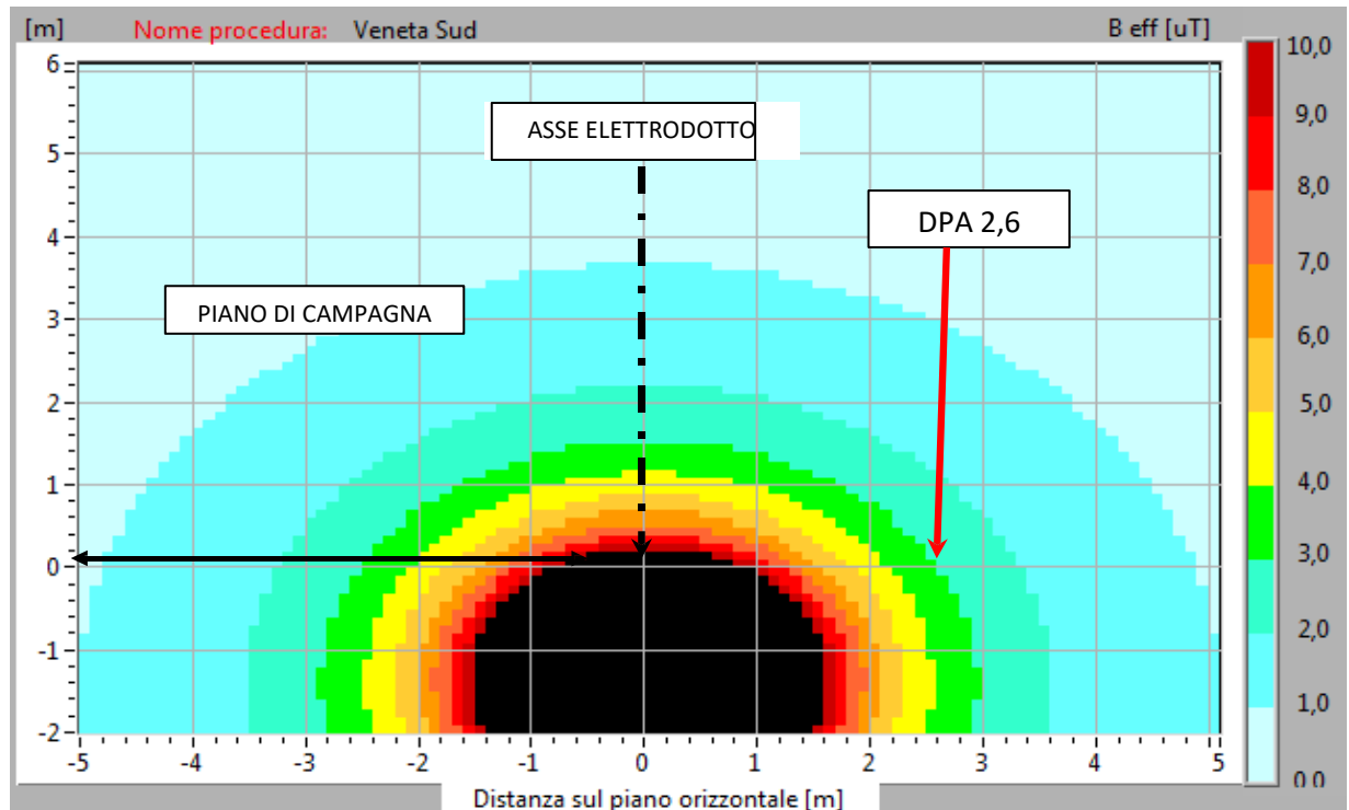
Figura 4 - Mapa verticale induzione magnetica (B) sezione tipo con indicazione della DPA - V=150\text{ kV} I = 900\text{ A}
