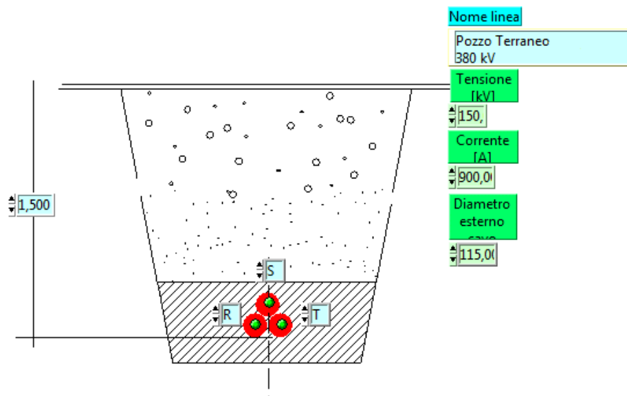
Figura 3 - Sezione tipo
